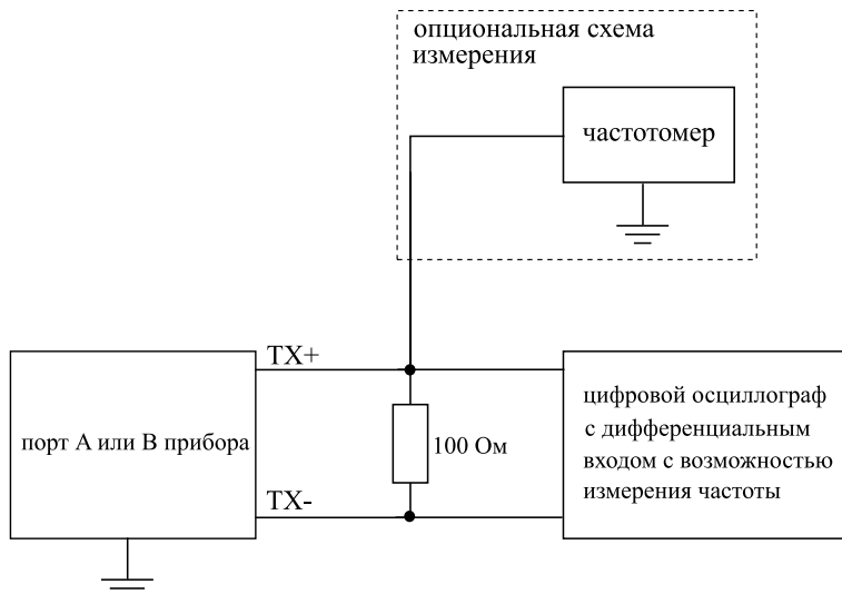
Рис. 15.1. Схема подключения
