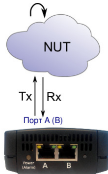
Рис. 3.7. Подключение прибора для тестирования с «А» на «А»
