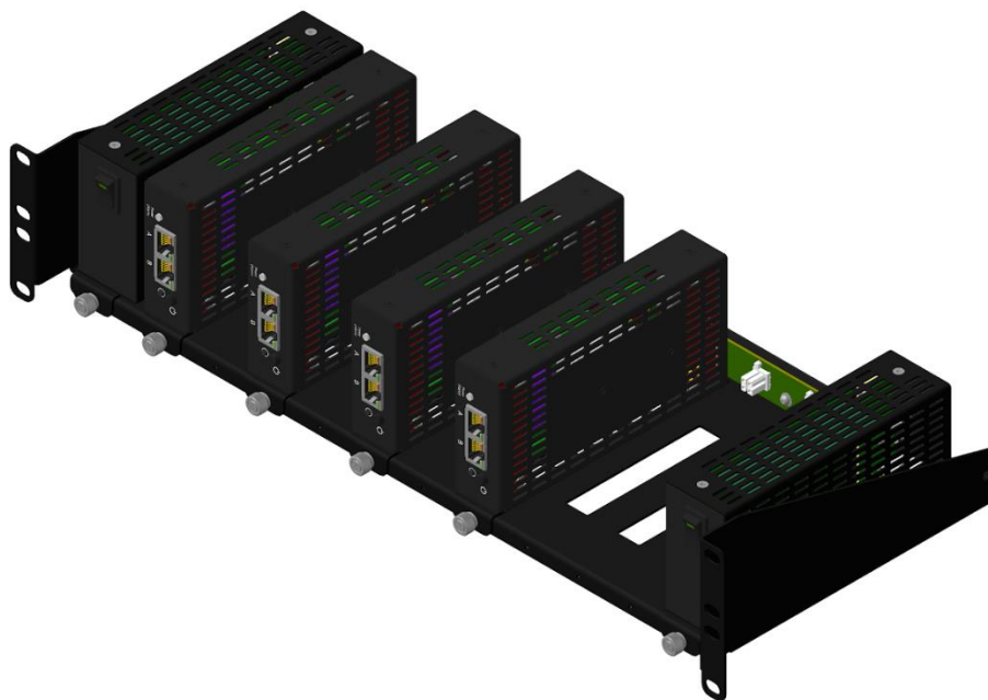
Рисунок 4.3. Неполное заполнение полки-шасси
