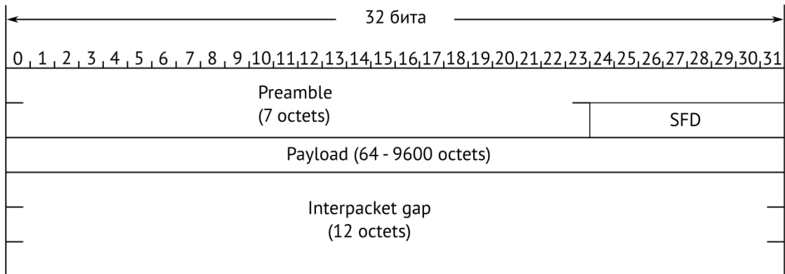
Рисунок 20.1. Структура пакета 1-го уровня
