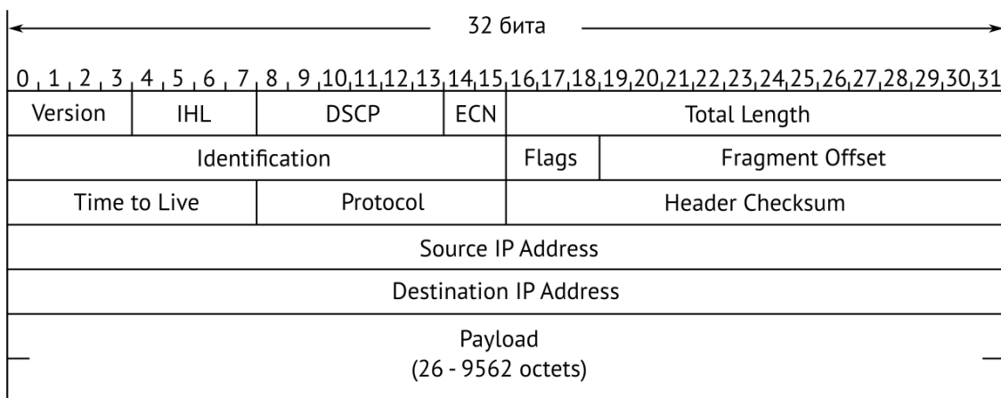
Рисунок 20.3. Структура пакета 3-го уровня
