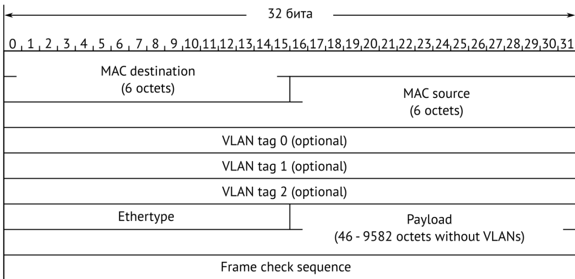
Рисунок 20.2. Структура кадра 2-го уровня
