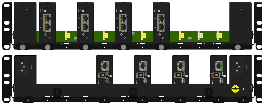
Рисунок 4.1. Установка приборов в полку-шасси
