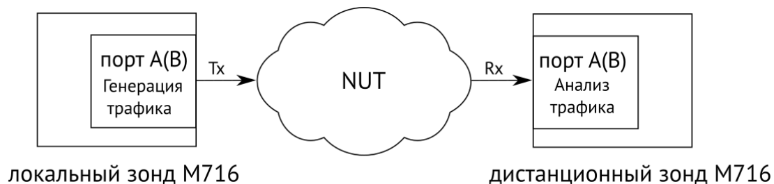
Рисунок 10.7. Схема однонаправленного теста
