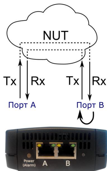
Рисунок 10.3. Подключение прибора для проведения измерений в двух направлениях
