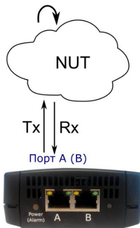
Рисунок 10.6. Подключение прибора для тестирования с «А» на «А»
