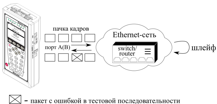
Рисунок 10.28. Тестирование на канальном/сетевом уровне (вариант 2)
