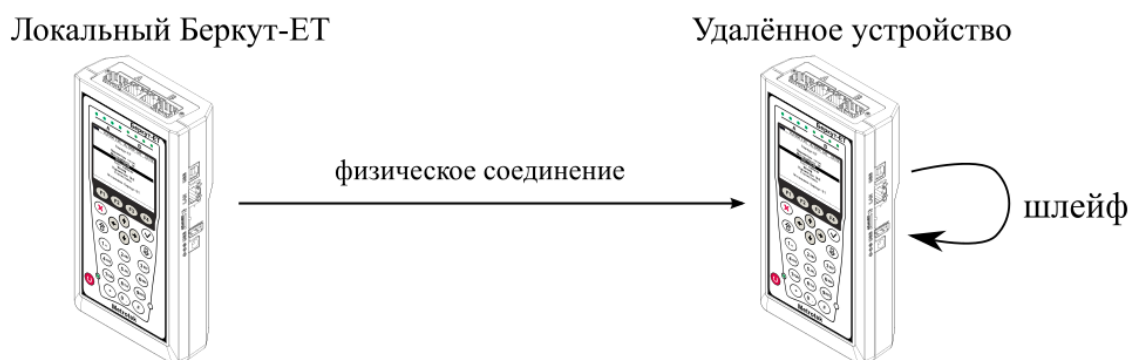
Рисунок 9.19. Схема тестирования
