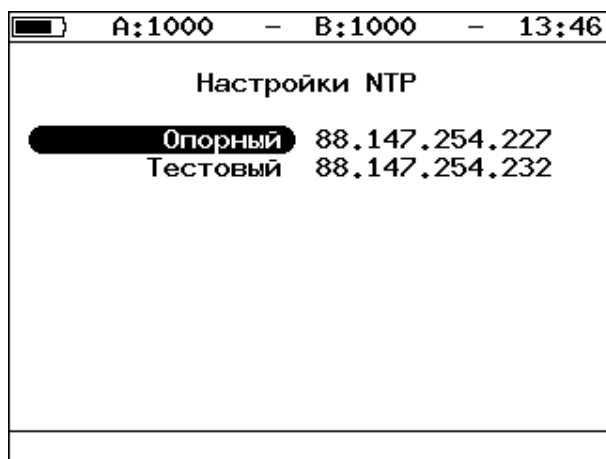
Рисунок 17.44. Меню «Настройки NTP»
