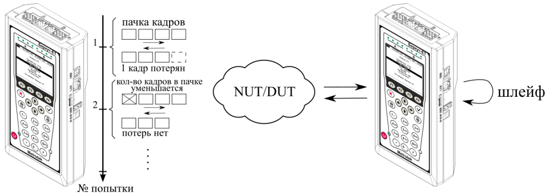
Рисунок 10.20. Анализ предельной нагрузки
