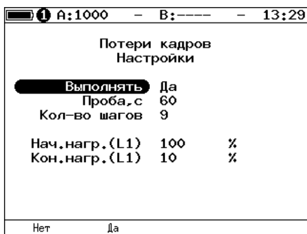
Рисунок 17.11. Настройка параметров теста
