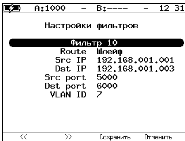
Рисунок 16.36. Сохранение или отмена настроек
