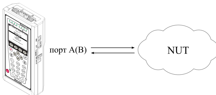
Рисунок 9.1. Вариант подключения 1
