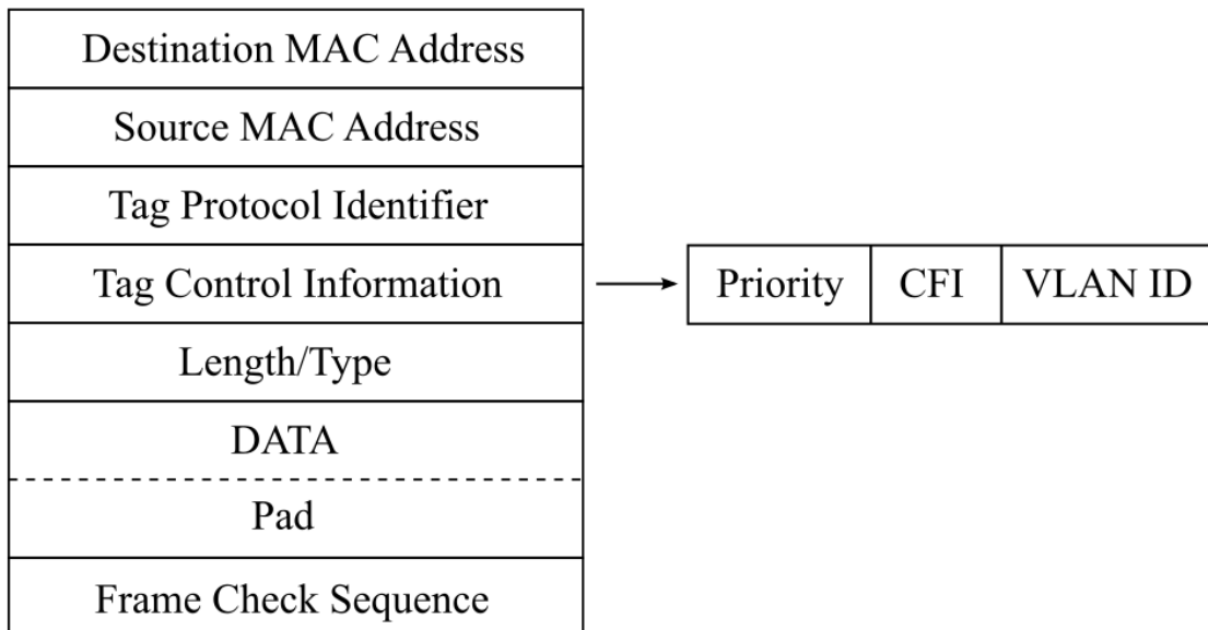
Рисунок 36.2. Структура Ethernet-кадра, содержащего VLAN-метку
