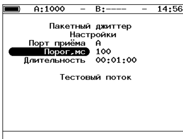
Рисунок 21.1. Меню «Пакетный джиттер. Настройки»
