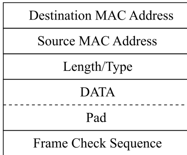
Рисунок 36.1. Структура Ethernet-кадра
