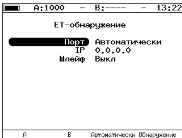
Рисунок 13.1. Меню «ET-обнаружение»
