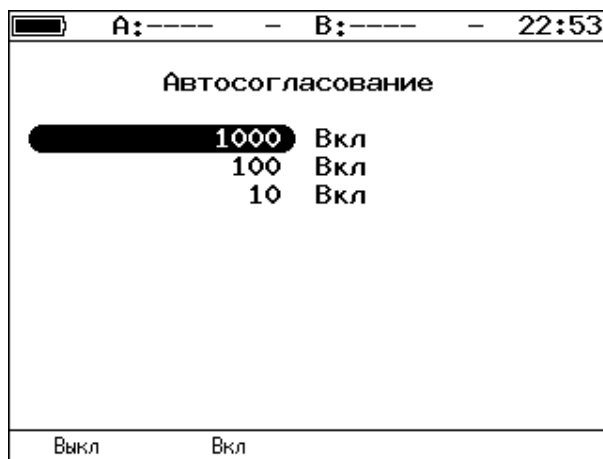
Рисунок 30.2. Меню «Автосогласование»
