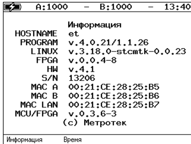
Рисунок 31.3. Экран «Информация»
