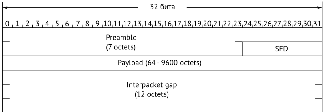
Рисунок 36.1. Структура пакета 1-го уровня
