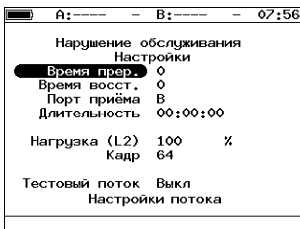
Рисунок 27.3. Меню «Настройки»
