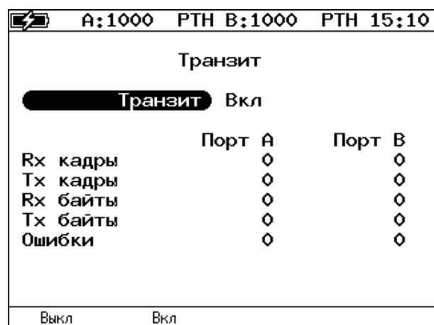
Рисунок 16.1. Меню «Транзит»
