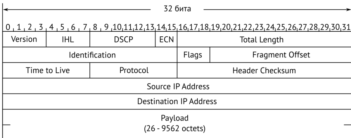
Рисунок 36.3. Структура пакета 3-го уровня
