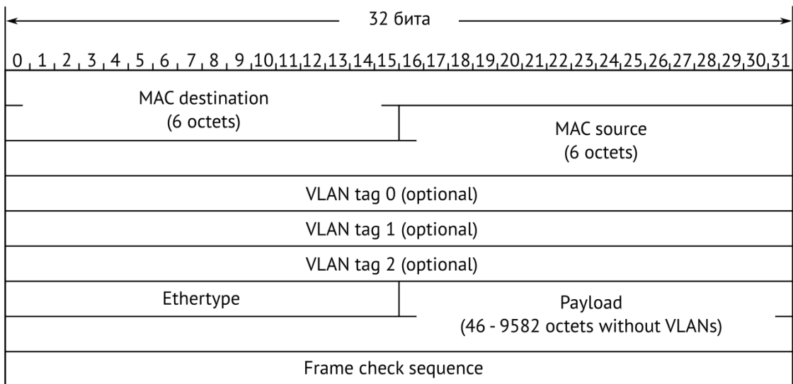
Рисунок 36.1. Структура пакета 1-го уровня
