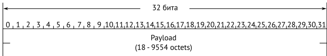
Рисунок 36.4. Структура дейтаграммы 4-го уровня
