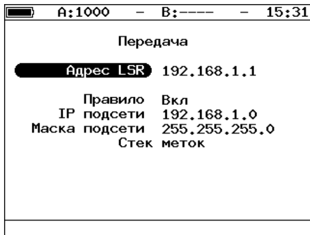
Рисунок 6.10. Меню «Передача»
