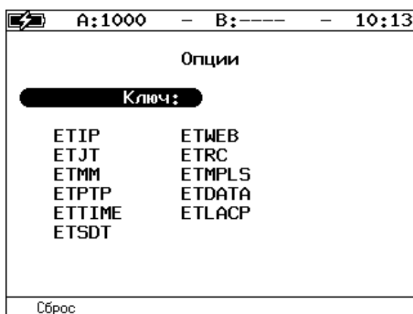
Рисунок 6.27. Меню «Опции»
