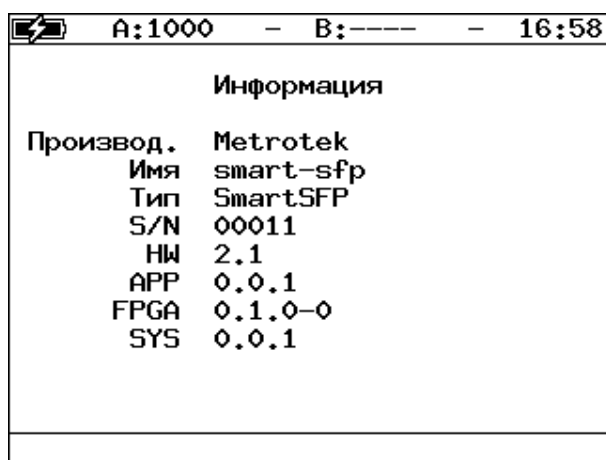
Рисунок 7.24. Меню «Информация»
