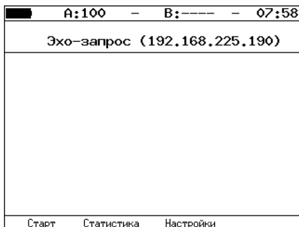
Рисунок 7.2. Меню «Эхо-запрос»
