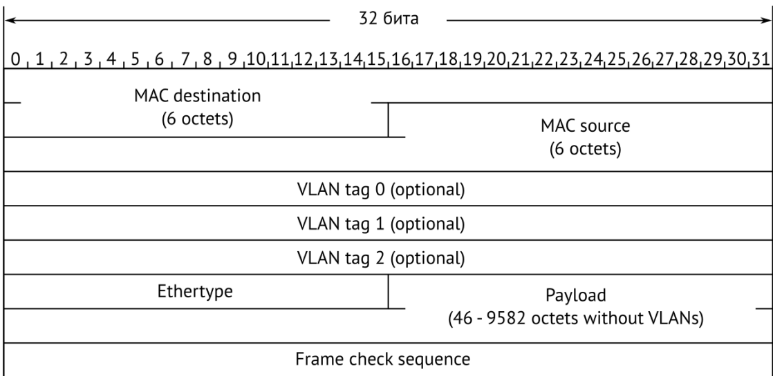
Рисунок 11.1. Структура пакета 1-го уровня
