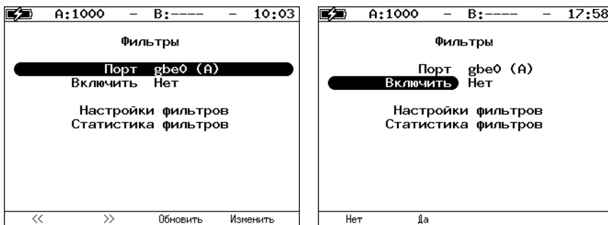
Рисунок 7.33. Меню «Фильтры»
