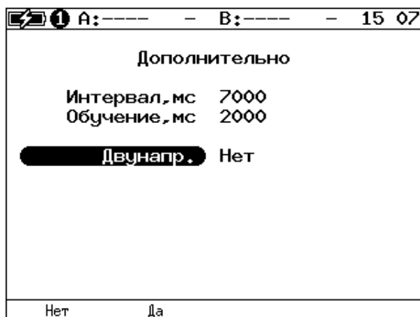
Рисунок 8.13. Меню «Дополнительно»
