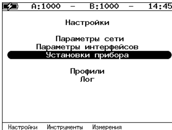
Рисунок 2.1. Меню «Настройки»
