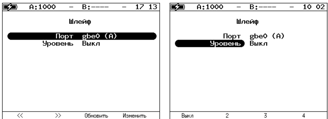
Рисунок 7.31. Меню «Шлейф»
