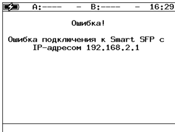
Рисунок 7.23. Ошибка подключения
