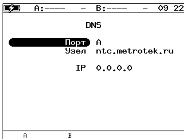
Рисунок 7.7. Меню «DNS»
