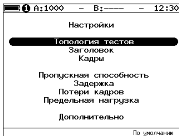
Рисунок 8.1. Настройки RFC 2544
