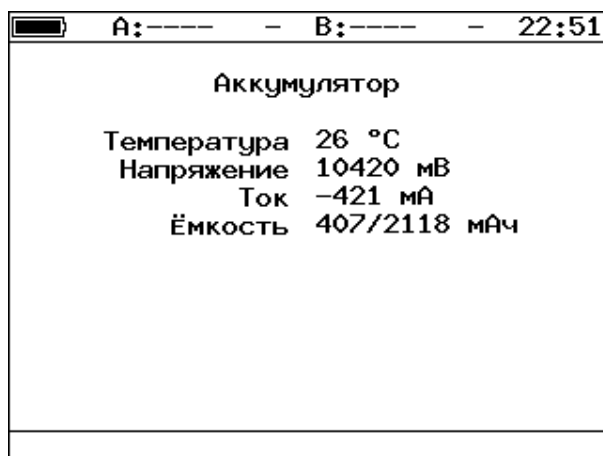
Рисунок 6.26. Экран «Аккумулятор»
