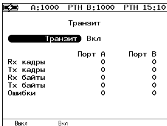
Рисунок 7.15. Меню «Транзит»
