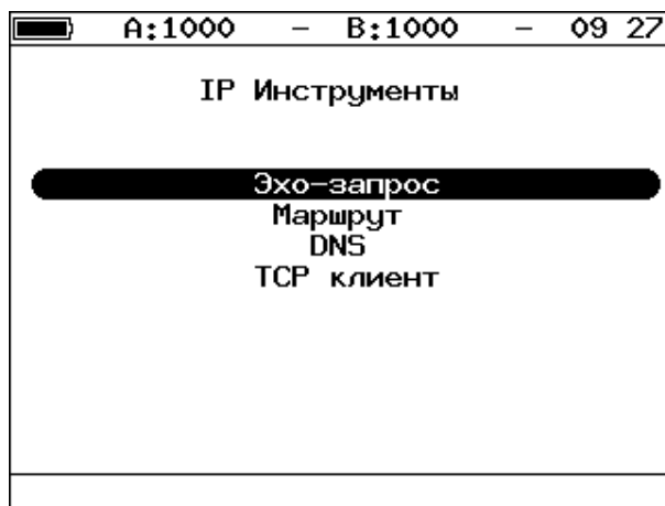
Рисунок 7.1. Меню «IP-инструменты»
