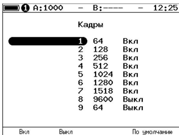
Рисунок 8.7. Меню «Кадры»
