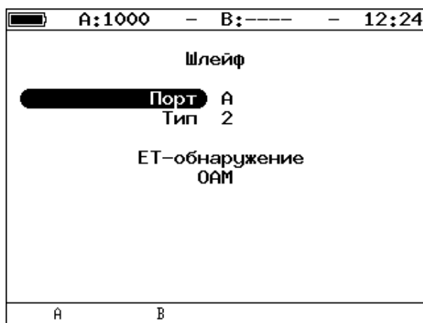
Рисунок 7.11. Меню «Шлейф»
