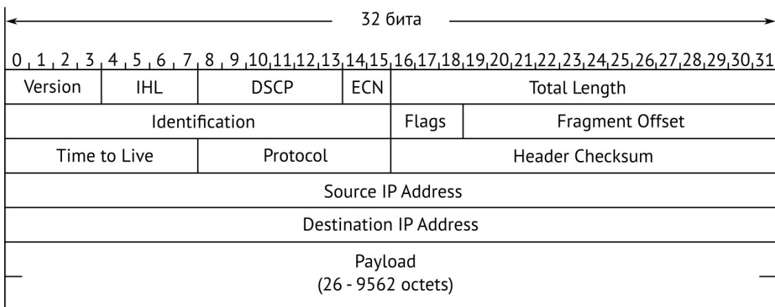
Рисунок 11.3. Структура пакета 3-го уровня
