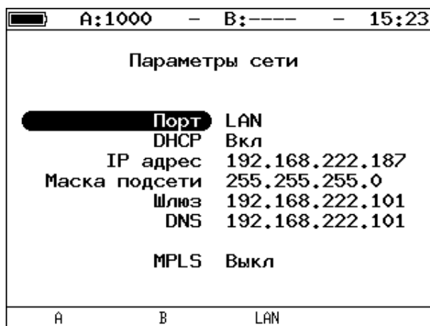
Рисунок 31.1. Меню «Параметры сети»
