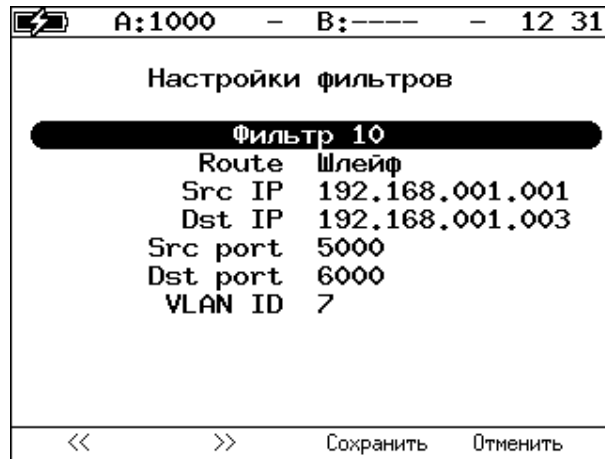
Рисунок 20.16. Сохранение или отмена настроек
