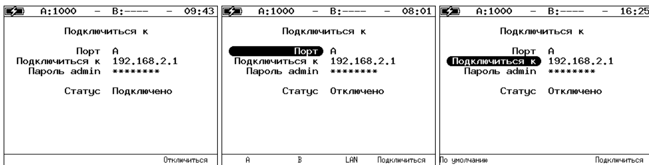
Рисунок 20.2. Меню «Подключиться к»
