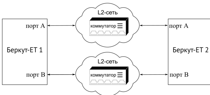
Рисунок 14.1. Подключение приборов для проведения мониторинга
