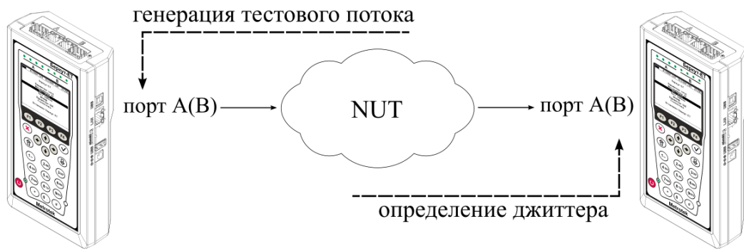
Рисунок 16.3. Измерение джиттера. Схема 3
