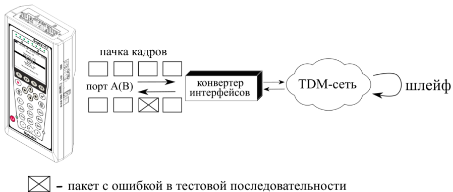
Рисунок 15.9. Тестирование на канальном/сетевом уровне (вариант 3)
