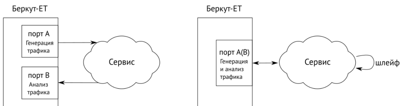
Рисунок 19.1. Схемы включения с использованием одного прибора
