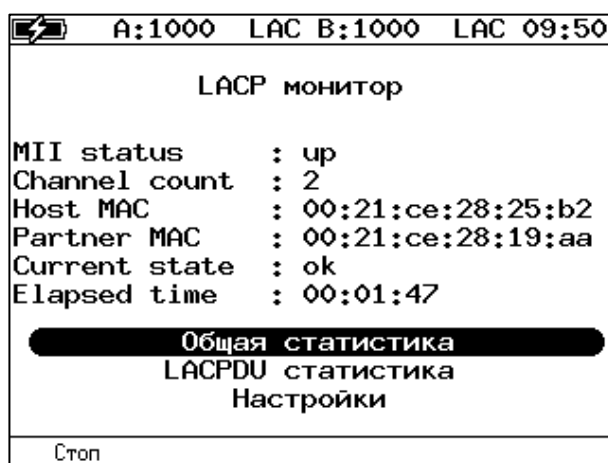
Рисунок 14.4. Меню «LACP монитор»
