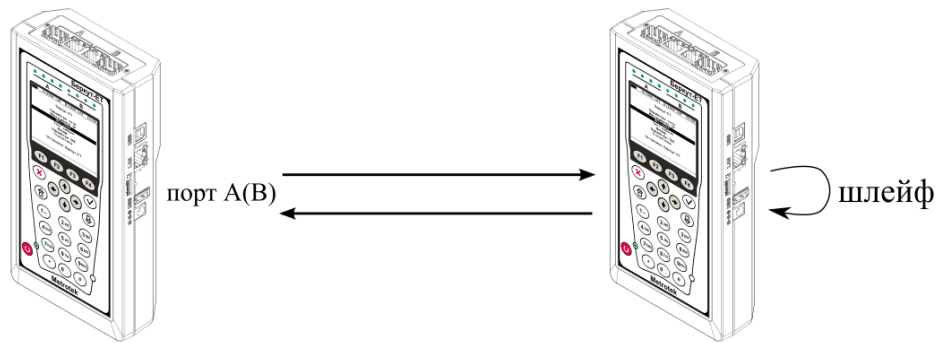
Рисунок 15.6. Тестирование на физическом уровне (вариант 2)
