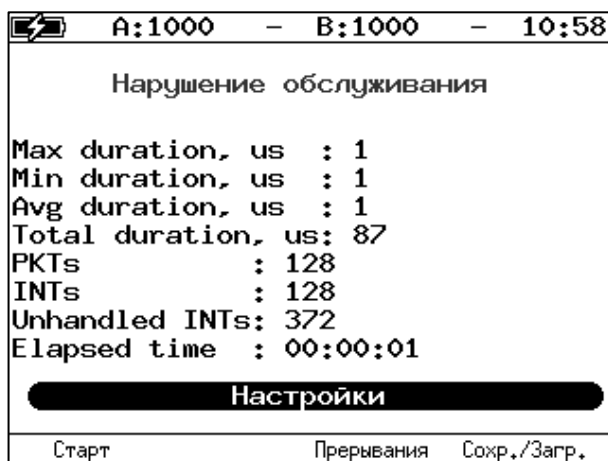
Рисунок 19.3. Пример результатов теста
