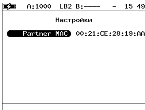
Рисунок 14.3. Настройки теста «LACP монитор»
