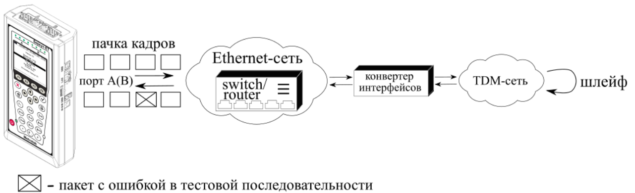
Рисунок 15.7. Тестирование на канальном/сетевом уровне (вариант 1)
