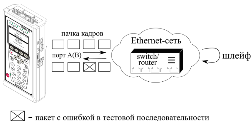
Рисунок 15.8. Тестирование на канальном/сетевом уровне (вариант 2)
