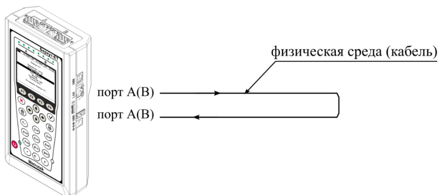
Рисунок 4.25. Тестирование на физическом уровне (вариант 1)
