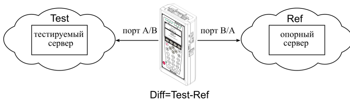
Рисунок 4.35. Типовая схема подключения для режима RTP
