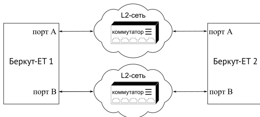
Рисунок 3.23. Подключение приборов для проведения мониторинга
