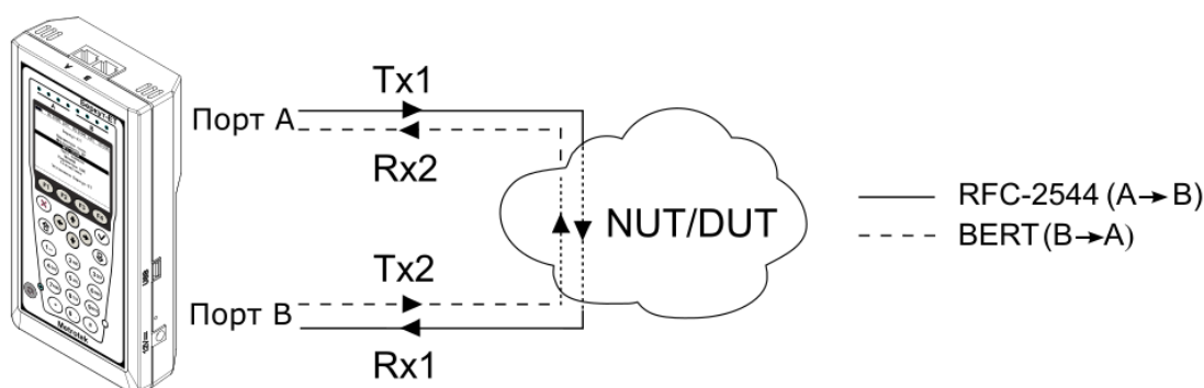
Рисунок 4.15. Схема параллельного тестирования: RFC-2544 и BERT
