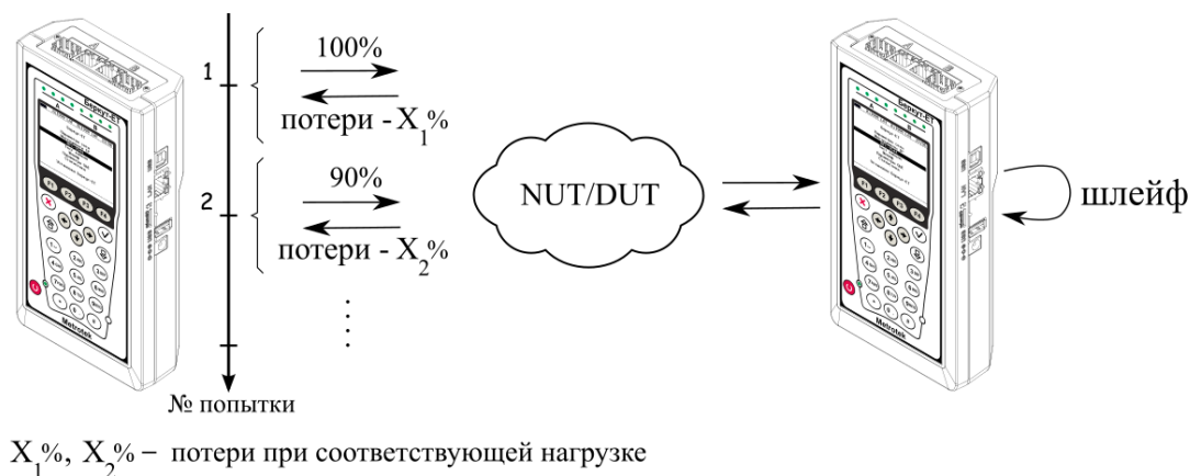
Рисунок 4.19. Анализ уровня потерь кадров
