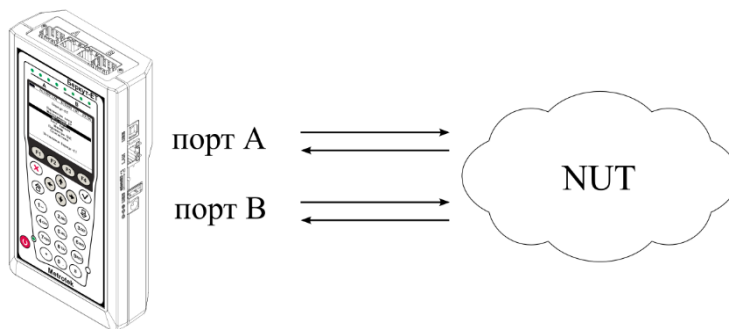
Рисунок 3.2. Вариант подключения 2
