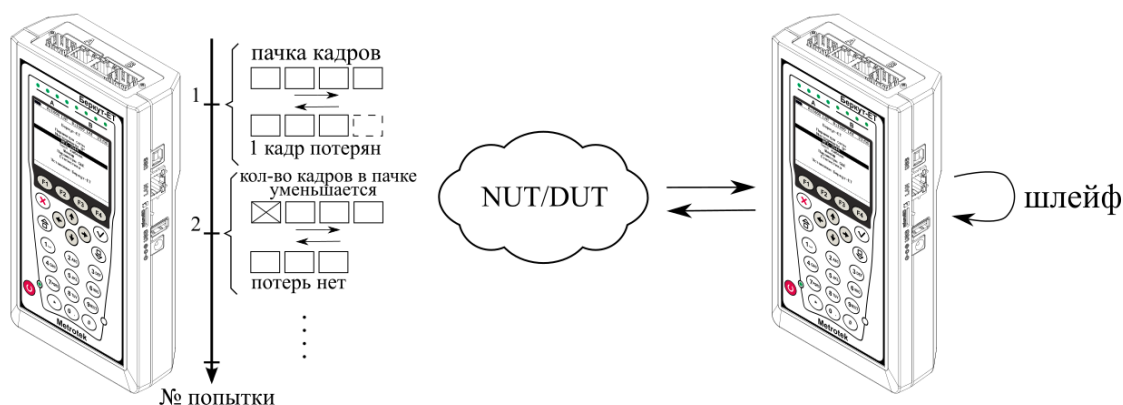
Рисунок 4.20. Анализ предельной нагрузки
