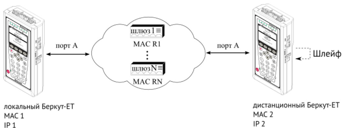
Рисунок 4.14. Типовая схема подключения
