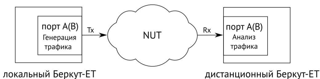
Рисунок 4.7. Схема однонаправленного теста
