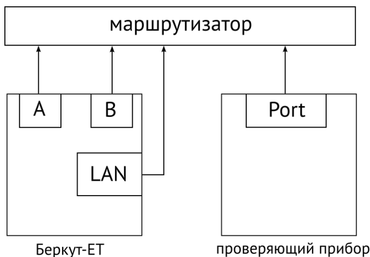
Рисунок 5.1. Схема подключения приборов для проверки выполнения требований по количеству переданной (принятой) информации
