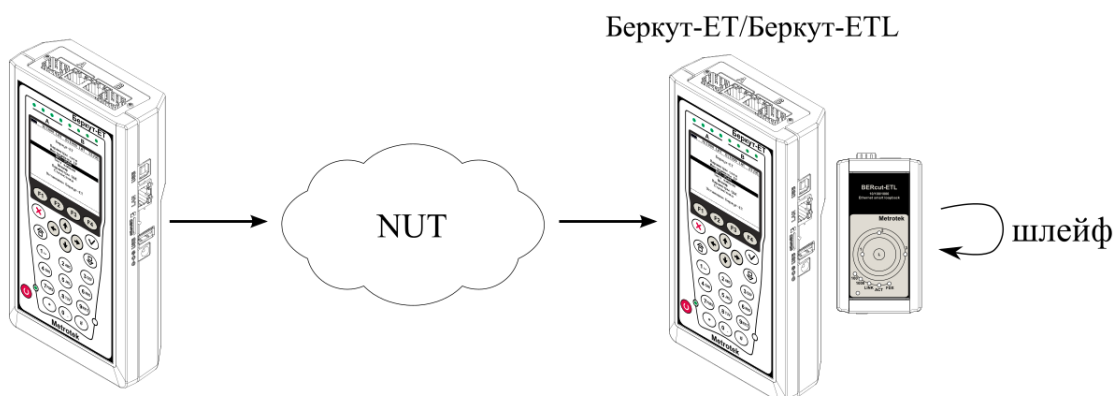
Рисунок 3.16. Схема тестирования
