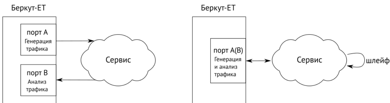
Рисунок 4.36. Схемы включения с использованием одного прибора
