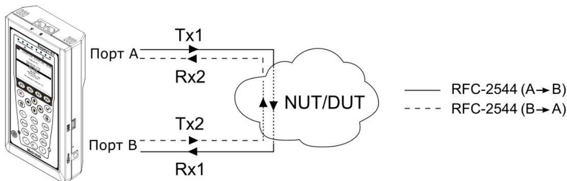
Рисунок 4.16. Схема двунаправленного теста RFC 2544
