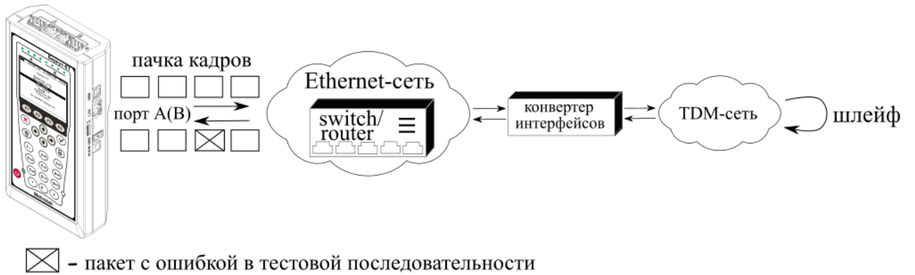
Рисунок 4.27. Тестирование на канальном/сетевом уровне (вариант 1)
