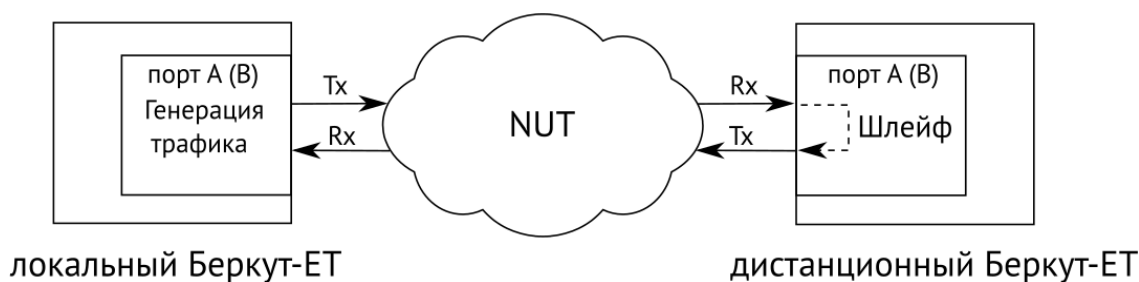
Рисунок 4.13. Схема двухнаправленного теста
