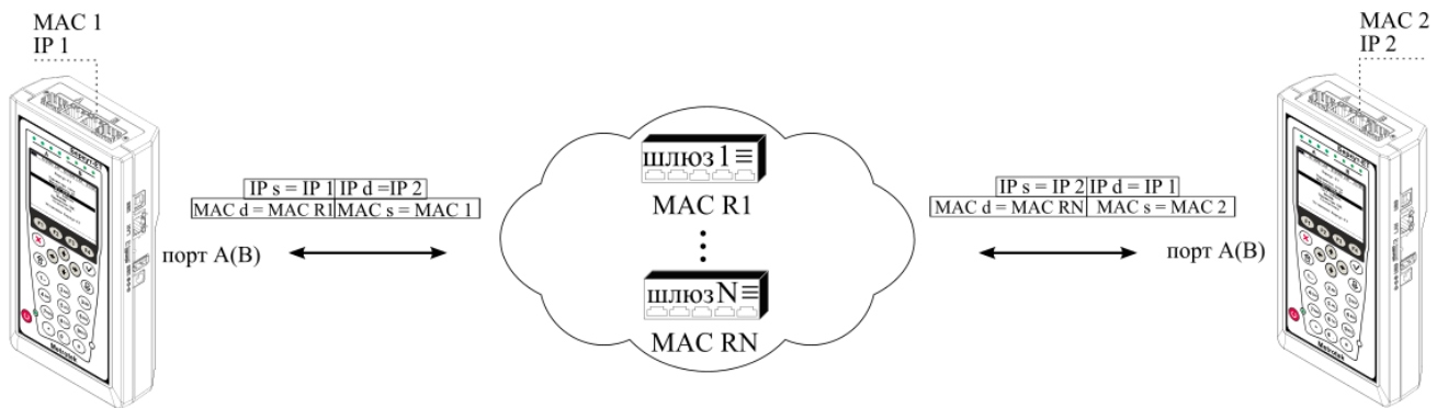
Рисунок 4.6. Типовая схема подключения 6
