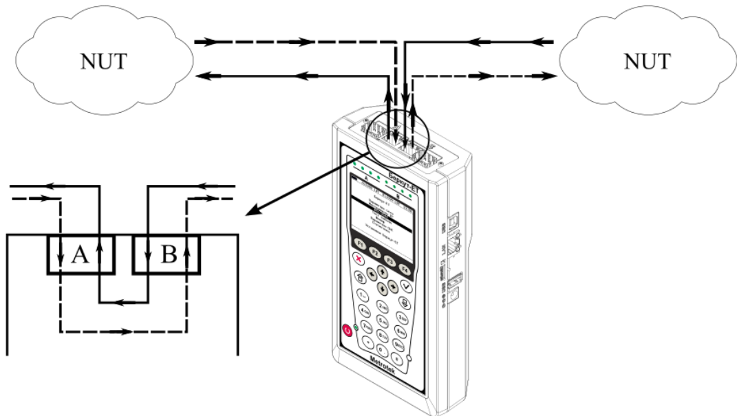
Рисунок 3.21. Пример подключения в режиме «Транзит»
