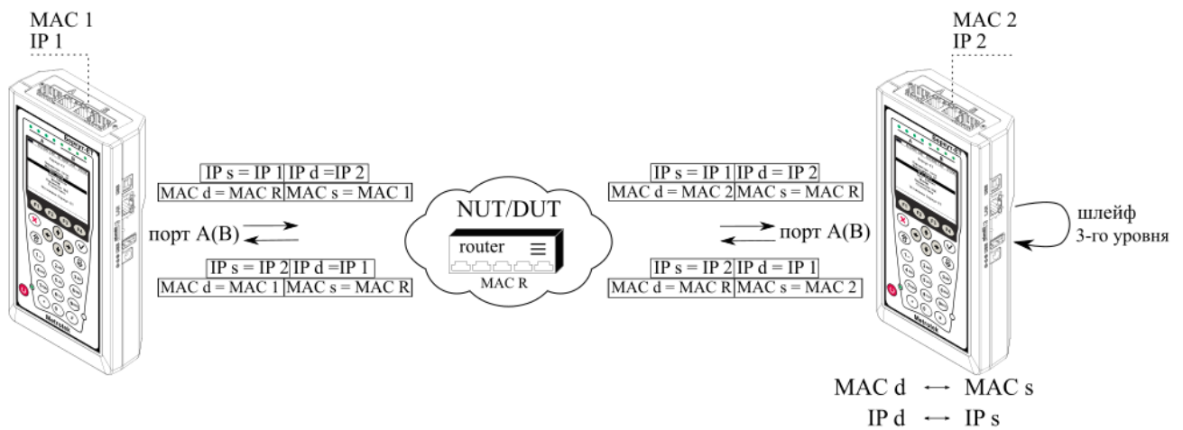
Рисунок 4.2. Типовая схема подключения 2
