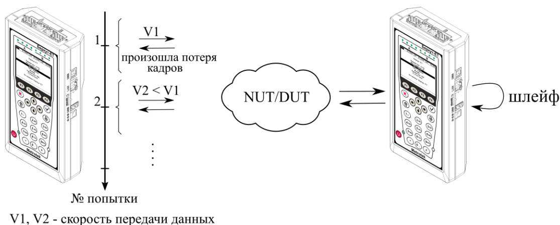
Рисунок 4.17. Анализ пропускной способности
