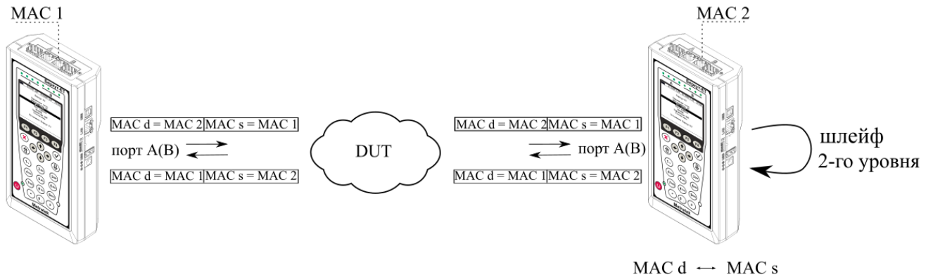
Рисунок 4.1. Типовая схема подключения 1
