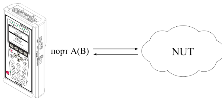
Рисунок 3.1. Вариант подключения 1
