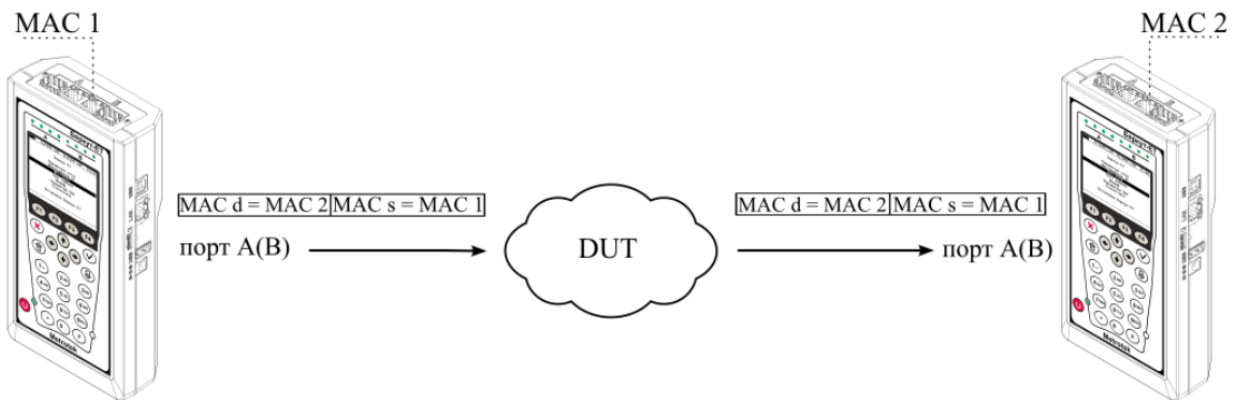
Рисунок 4.5. Типовая схема подключения 5
