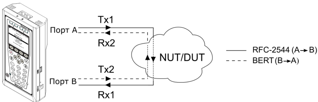
Рисунок 8.1. Схема параллельного тестирования: RFC-2544 и BERT
