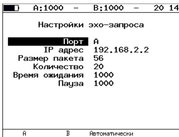
Рисунок 11.4. Меню «Настройки эхо-запроса»
