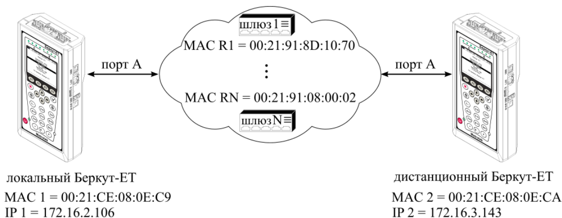
Рисунок 8.4. Типовая схема подключения
