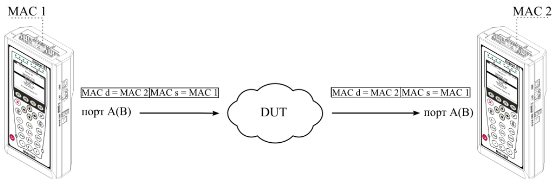
Рисунок 7.5. Типовая схема подключения 5
