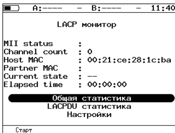
Рисунок 15.2. Меню «LACP монитор»
