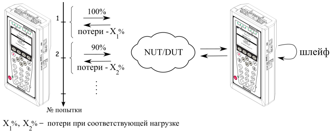
Рисунок 3.3. Анализ уровня потерь кадров
