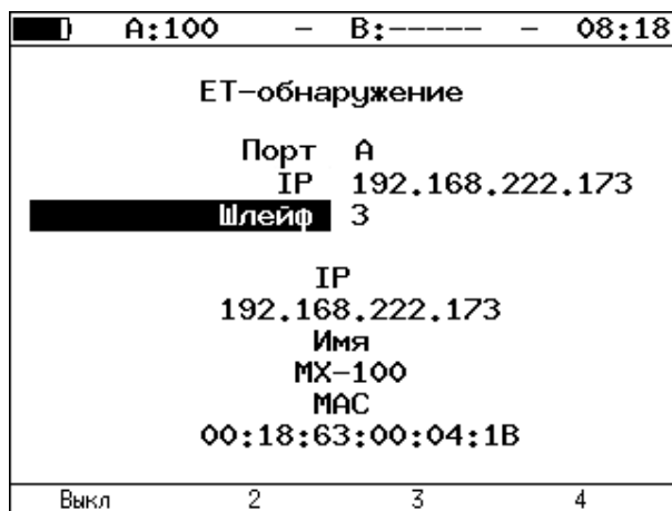
Рисунок 10.3. Пример выполнения ET-обнаружения
