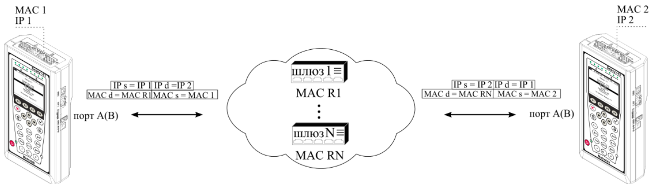
Рисунок 7.6. Типовая схема подключения 6
