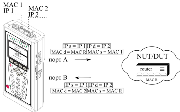
Рисунок 7.3. Типовая схема подключения 3
