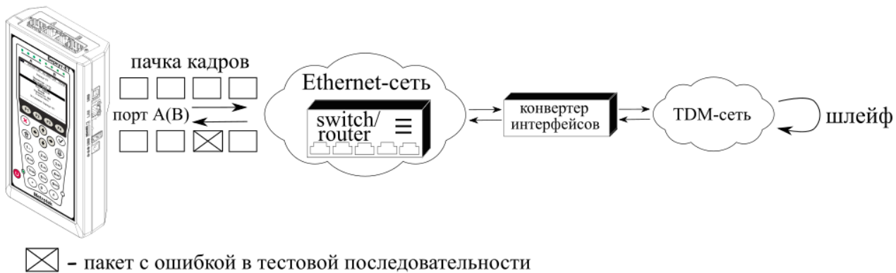
Рисунок 16.7. Тестирование на канальном/сетевом уровне (вариант 1)
