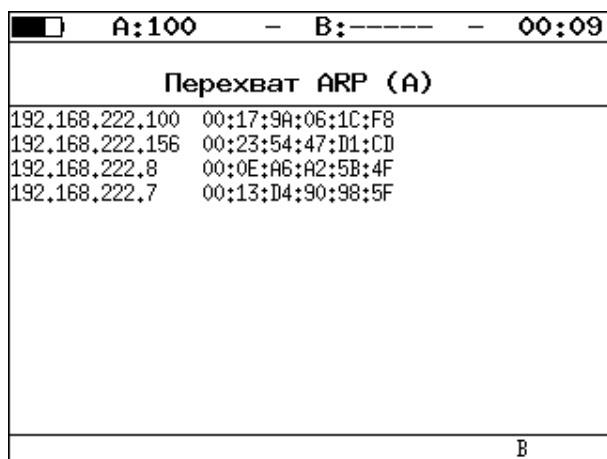
Рисунок 12.2. Экран «ARP монитор»
