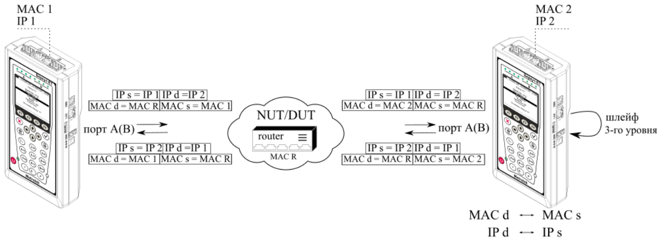
Рисунок 7.2. Типовая схема подключения 2
