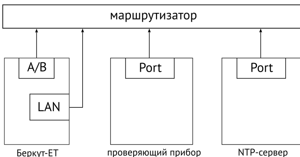
Рисунок 21.2. Схема подключения приборов для проверки выполнения требований по расхождению шкалы времени
