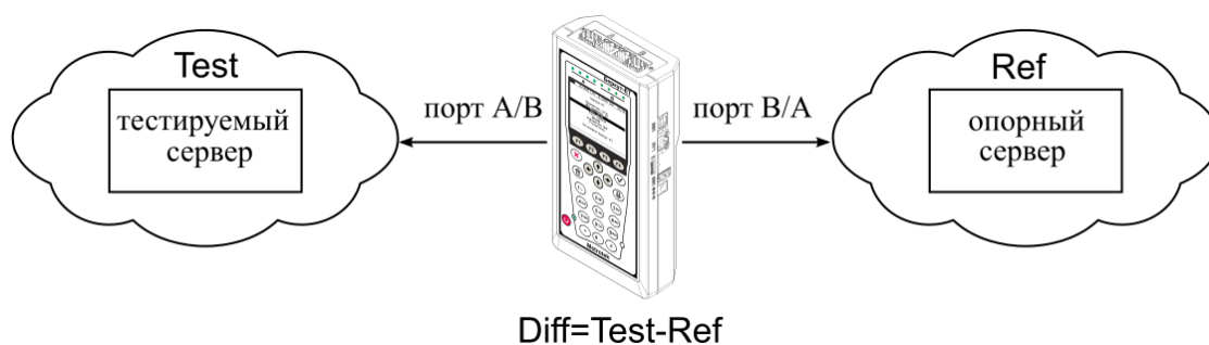
Рисунок 18.2. Типовая схема подключения для режима RTP
