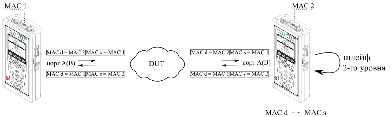
Рисунок 7.1. Типовая схема подключения 1
