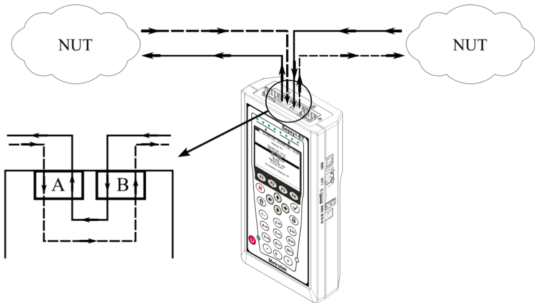
Рисунок 13.1. Пример подключения в режиме «Транзит»
