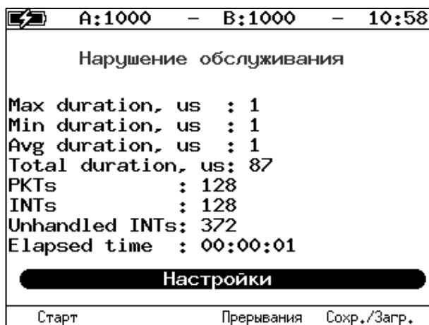
Рисунок 20.3. Пример результатов теста
