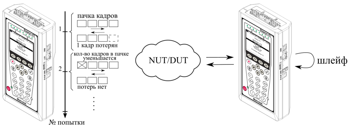
Рисунок 3.4. Анализ предельной нагрузки
