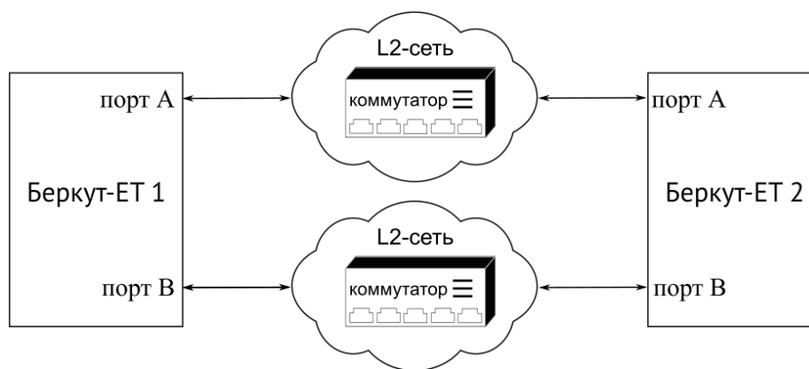
Рисунок 15.1. Подключение приборов для проведения мониторинга
