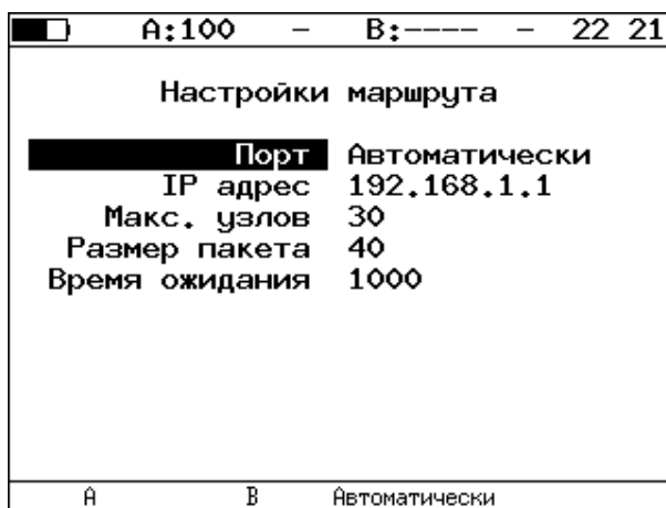
Рисунок 11.8. Меню «Настройки маршрута»
