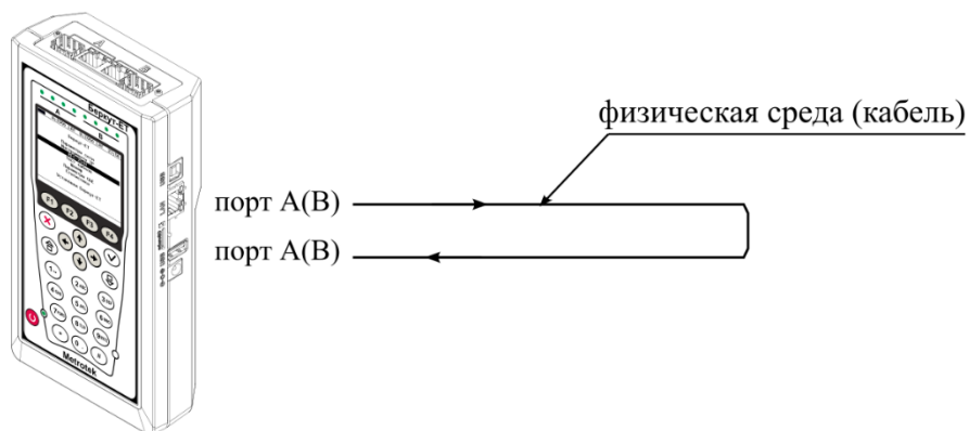
Рисунок 16.5. Тестирование на физическом уровне (вариант 1)
