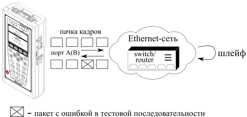
Рисунок 16.8. Тестирование на канальном/сетевом уровне (вариант 2)
