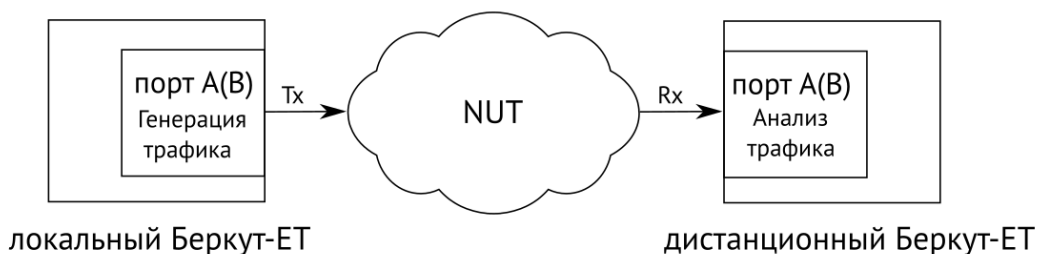
Рисунок 8.3. Схема однонаправленного теста
