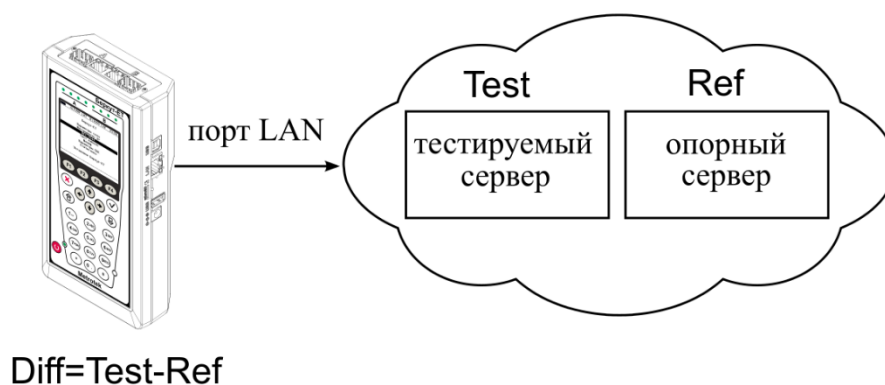
Рисунок 18.1. Типовая схема подключения для режима NTP
