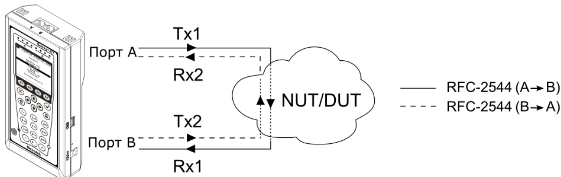
Рисунок 8.2. Схема двунаправленного теста RFC 2544
