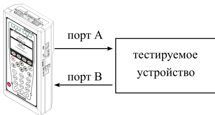
Рисунок 19.1. Типовая схема подключения для проведения теста «Тестовые данные»
