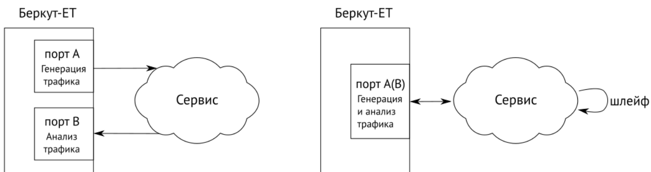
Рисунок 20.1. Схемы включения с использованием одного прибора
