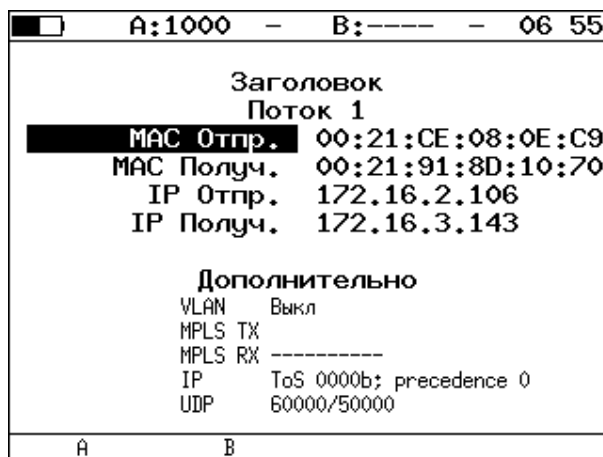
Рисунок 10.3. Экран «Заголовок»
