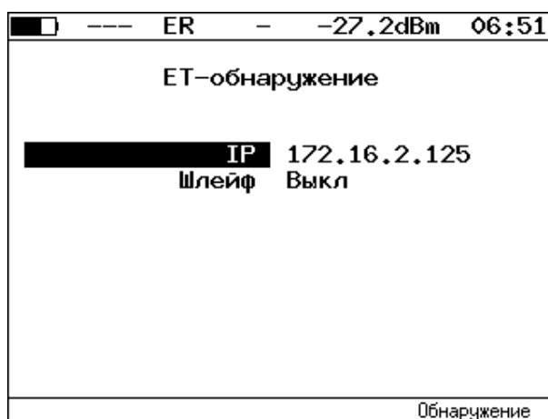
Рисунок 14.2. Меню «ET-обнаружение»
