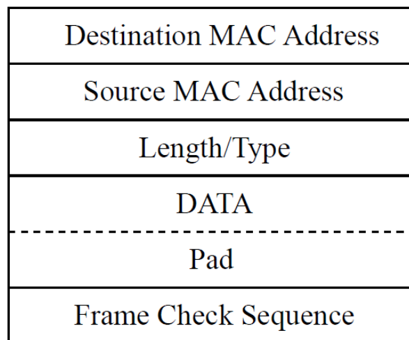
Рисунок 32.1. Структура Ethernet-кадра
