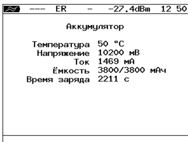
Рисунок 24.4. Экран «Аккумулятор»
