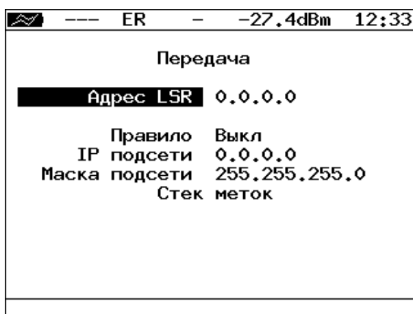
Рисунок 23.4. Меню «Передача»
