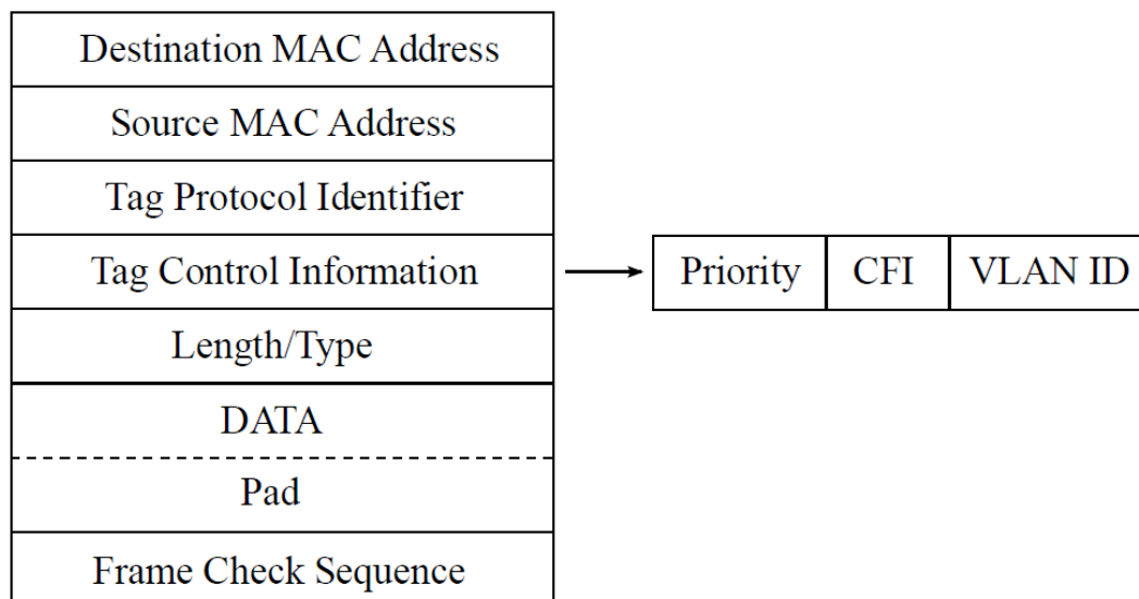
Рисунок 32.2. Структура Ethernet-кадра, содержащего VLAN-метку
