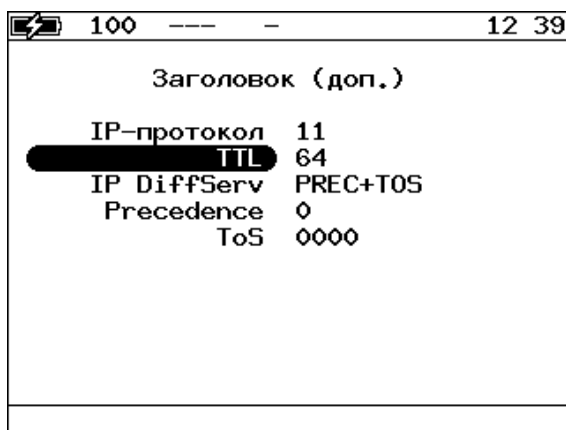
Рисунок 7.6. Настройка IP
