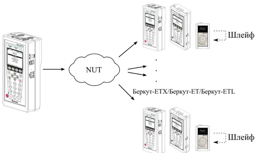
Рисунок 14.1. Схема тестирования
