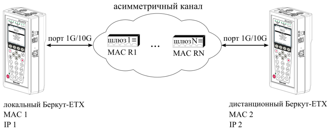
Рисунок 10.2. Типовая схема подключения
