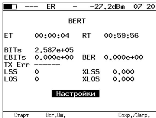
Рисунок 17.5. Экран «BERT»
