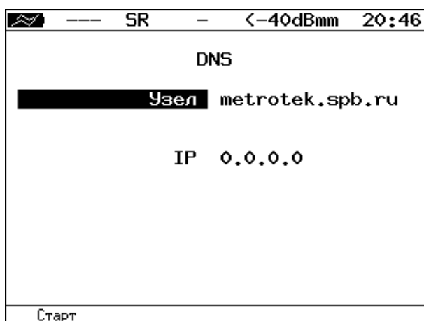
Рисунок 15.9. Меню «DNS»
