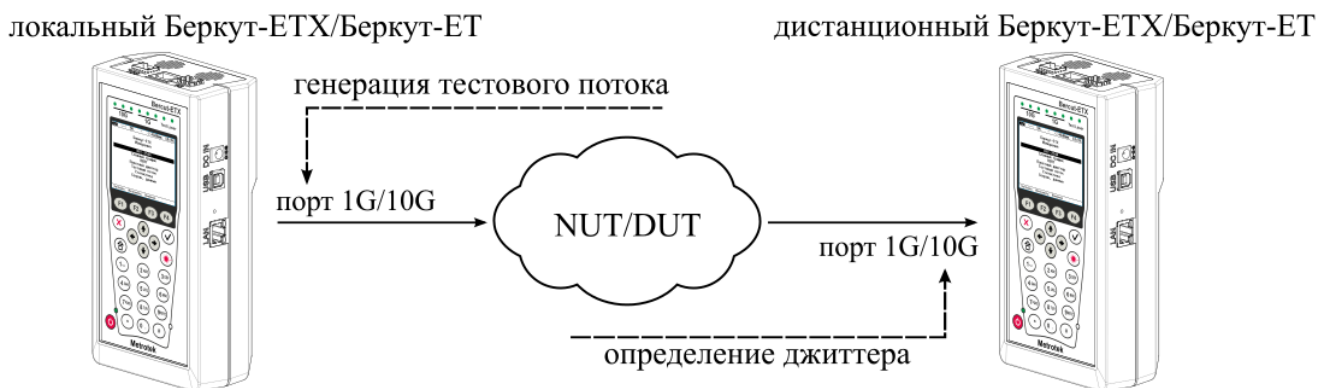
Рисунок 19.3. Генерация постоянного трафика. Схема 2
