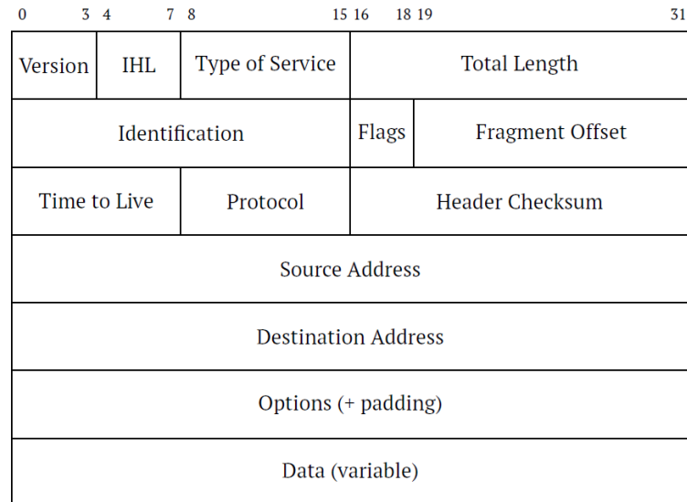
Рисунок 31.1. Структура пакета IPv4
