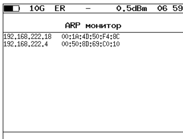
Рисунок 15.11. Результаты тестирования
