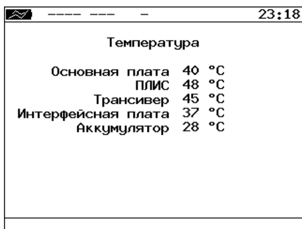
Рисунок 24.5. Меню «Температура»
