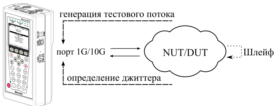
Рисунок 19.2. Генерация постоянного трафика. Схема 1
