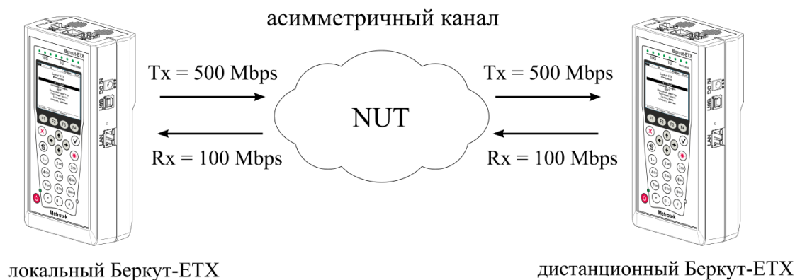
Рисунок 10.1. Пример асимметричного канала
