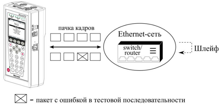
Рисунок 17.11. Тестирование на канальном/сетевом уровне (вариант 2)
