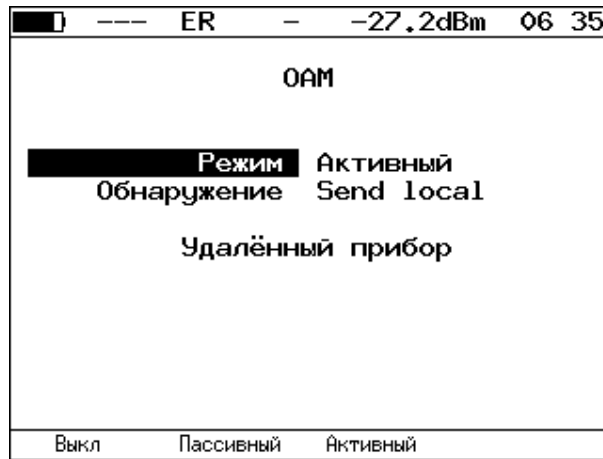
Рисунок 13.2. Меню «OAM»
