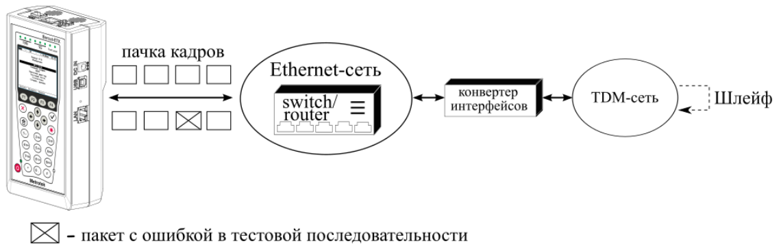
Рисунок 17.10. Тестирование на канальном/сетевом уровне (вариант 1)
