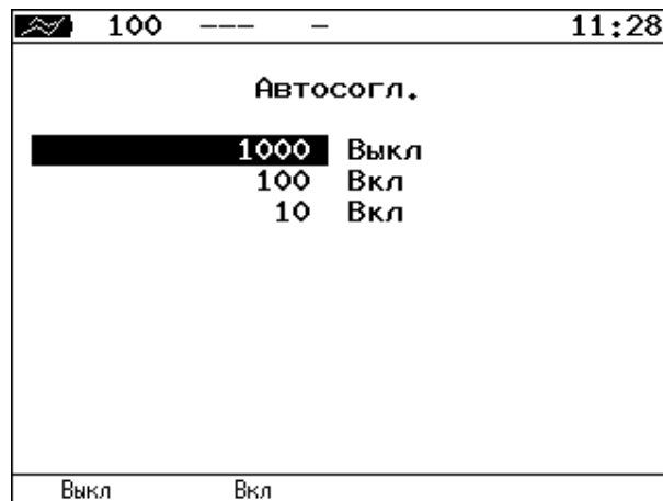
Рисунок 23.2. Меню «Автосогласование»
