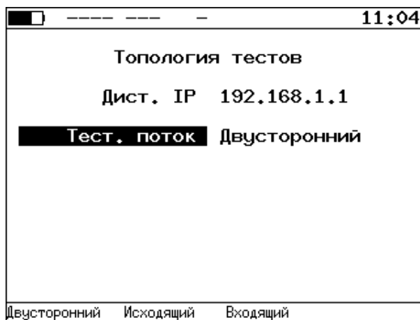
Рисунок 7.3. Меню «Топология»
