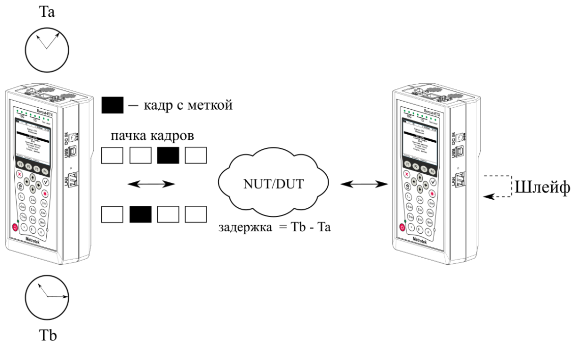
Рисунок 6.2. Анализ задержки
