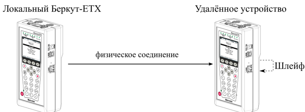
Рисунок 13.1. Схема тестирования
