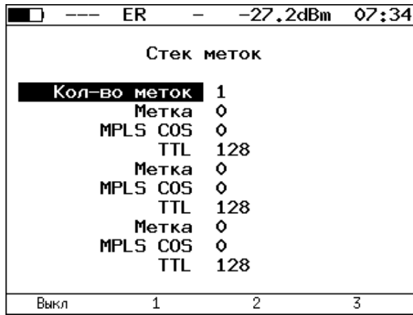
Рисунок 17.7. Меню «MPLS»
