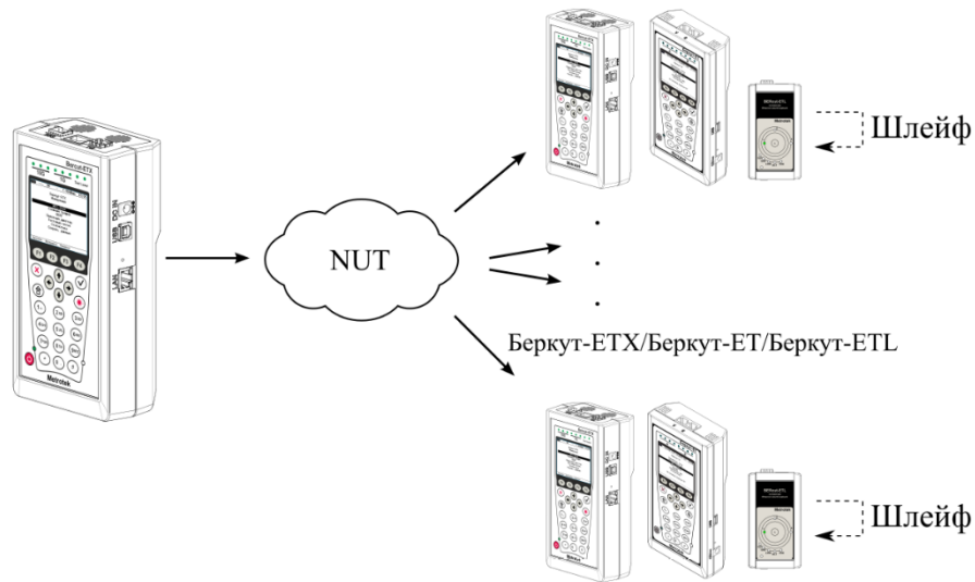
Рисунок 14.1. Схема тестирования
