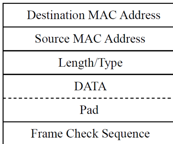
Рисунок 32.1. Структура Ethernet-кадра
