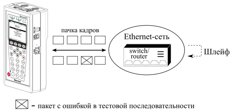
Рисунок 17.11. Тестирование на канальном/сетевом уровне (вариант 2)
