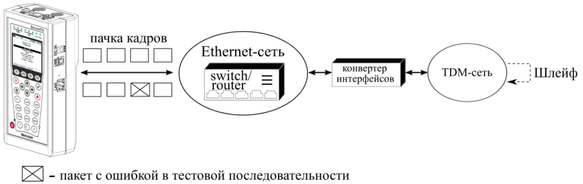
Рисунок 9.63. Тестирование на канальном/сетевом уровне (вариант 1)
