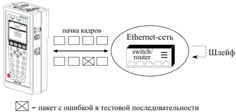
Рисунок 9.64. Тестирование на канальном/сетевом уровне (вариант 2)
