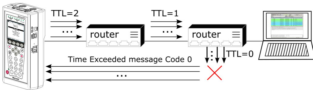
Рисунок 9.21. Проверка устойчивости маршрутизатора к приёму пакетов с TTL=0
