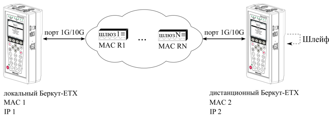
Рисунок 9.7. Типовая схема подключения
