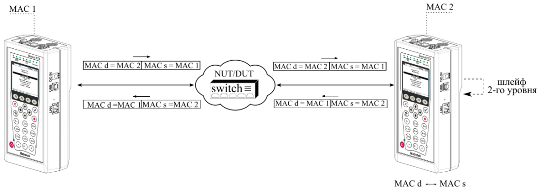
Рисунок 9.1. Типовая схема подключения 1
