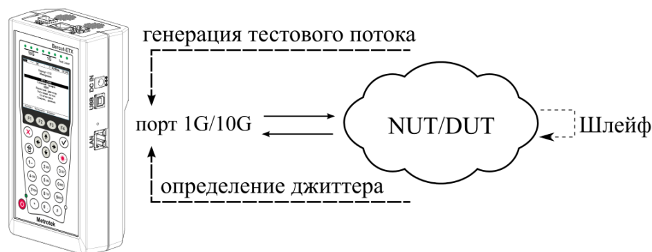
Рисунок 9.72. Генерация постоянного трафика. Схема 1
