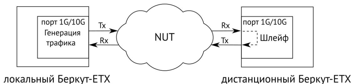
Рисунок 9.6. Схема двунаправленного теста
