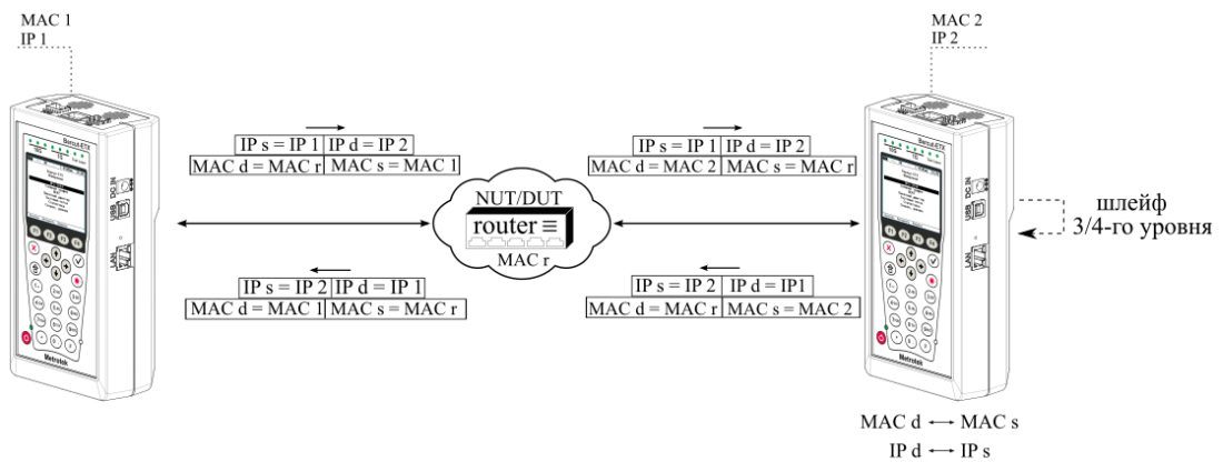
Рисунок 9.2. Типовая схема подключения 2
