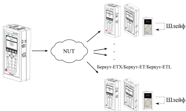
Рисунок 8.17. Схема тестирования
