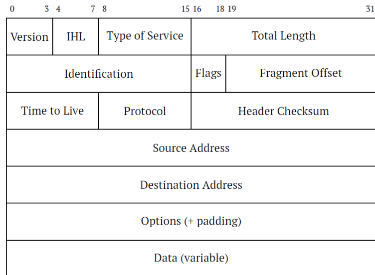
Рисунок 15.1. Структура пакета IPv4
