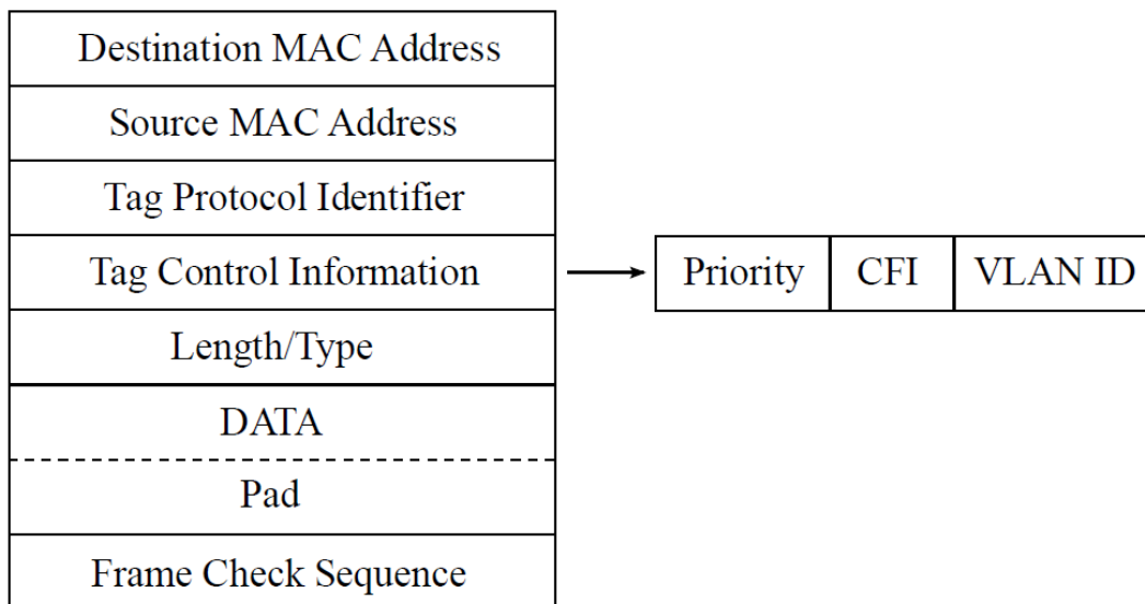
Рисунок 16.2. Структура Ethernet-кадра, содержащего VLAN-метку
