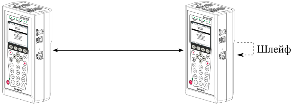
Рисунок 9.62. Тестирование на физическом уровне (вариант 2)
