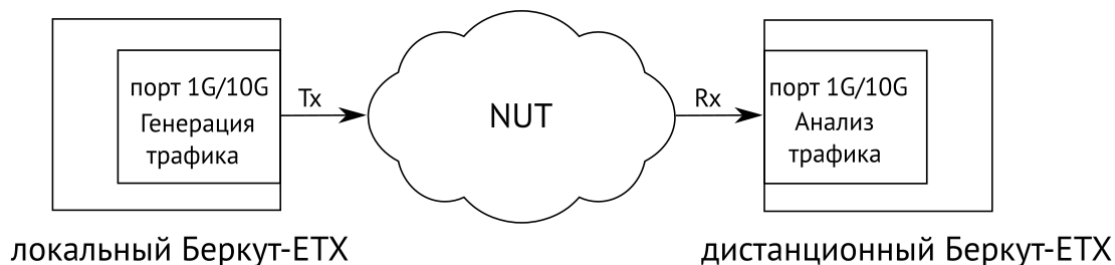
Рисунок 9.9. Схема однонаправленного теста
