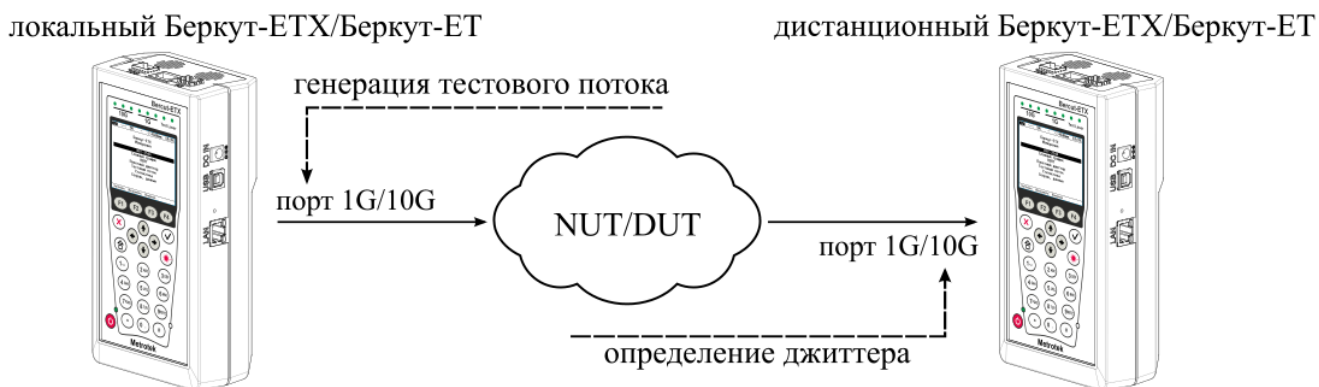
Рисунок 9.73. Генерация постоянного трафика. Схема 2
