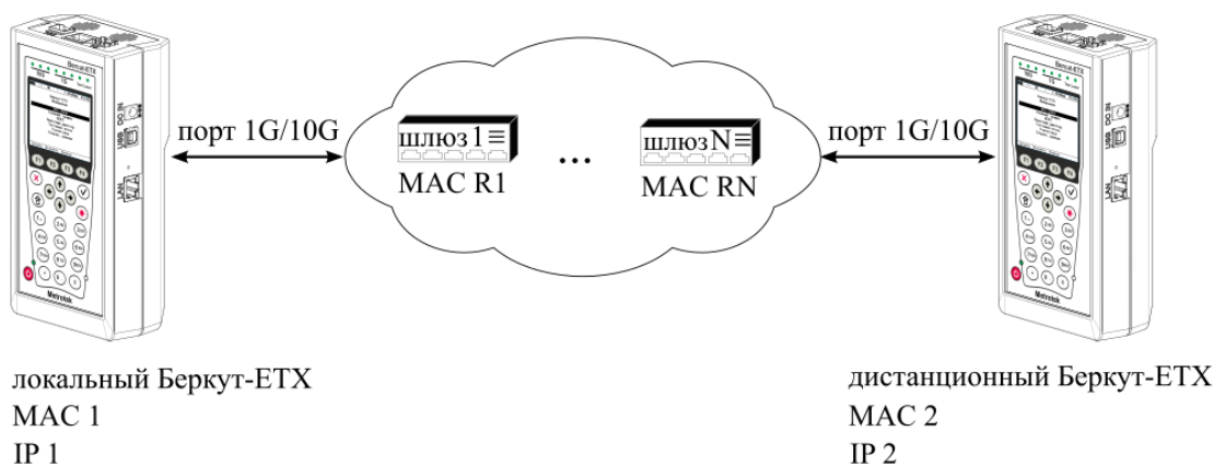
Рисунок 9.10. Типовая схема подключения
