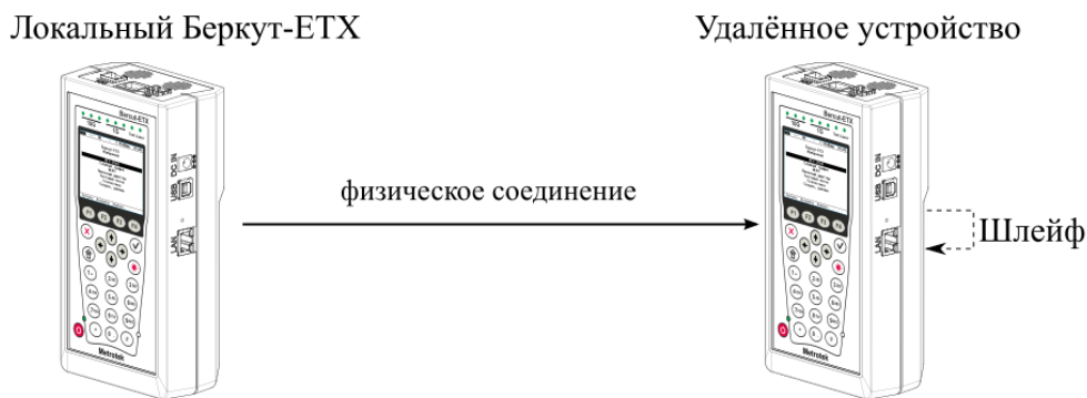
Рисунок 8.20. Схема тестирования
