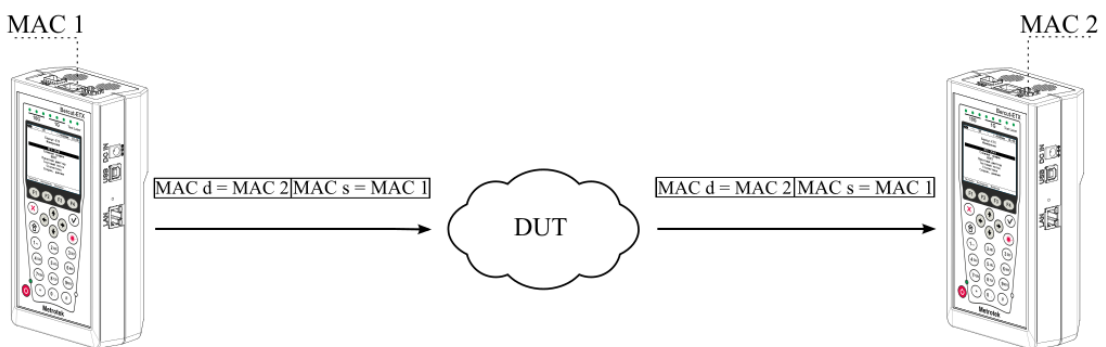
Рисунок 9.3. Типовая схема подключения 3
