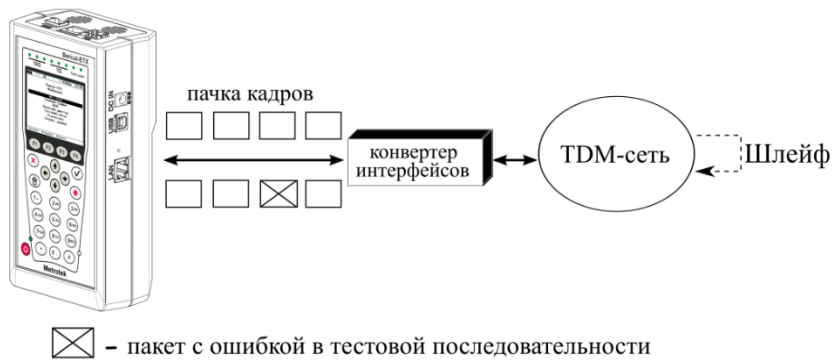
Рисунок 9.65. Тестирование на канальном/сетевом уровне (вариант 3)
