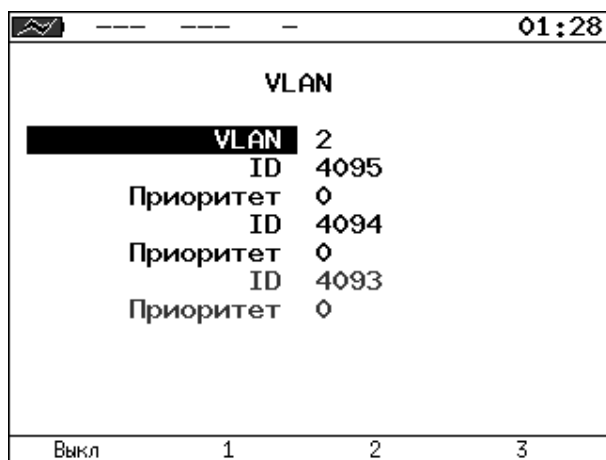
Рисунок 6.4. Меню «VLAN»
