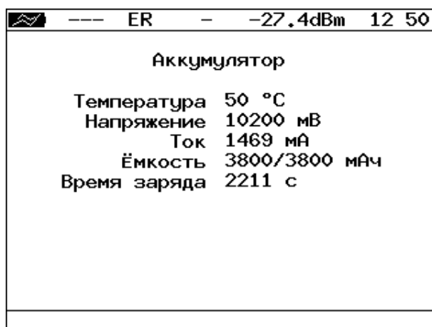
Рисунок 6.15. Экран «Аккумулятор»
