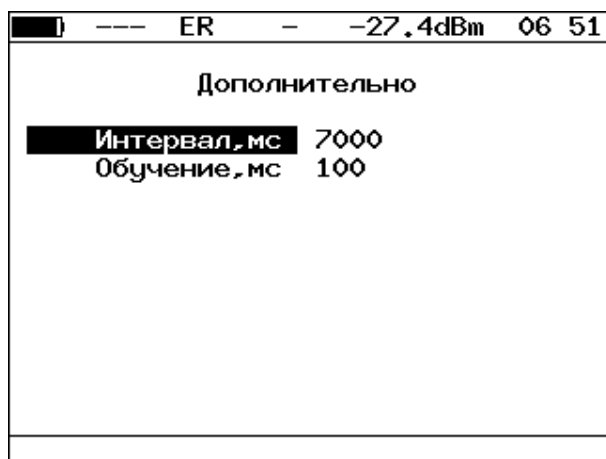
Рисунок 9.29. Меню «Дополнительно»
