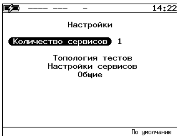
Рисунок 9.46. Меню «Настройки»
