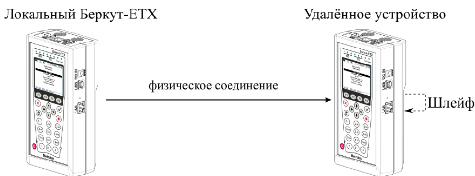
Рисунок 8.20. Схема тестирования
