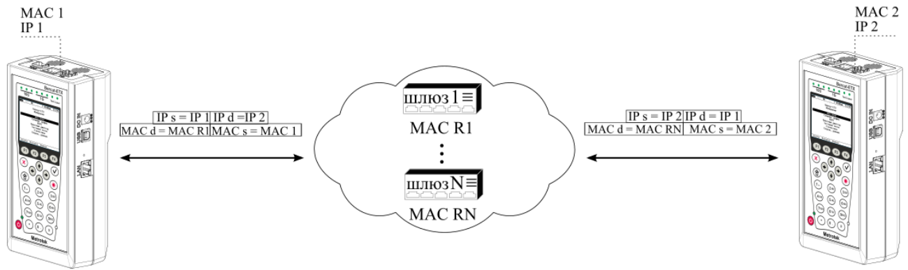
Рисунок 9.4. Типовая схема подключения 4
