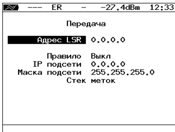
Рисунок 6.6. Меню «Передача»
