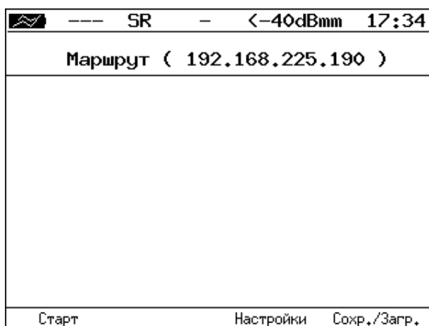
Рисунок 8.6. Меню «Маршрут»
