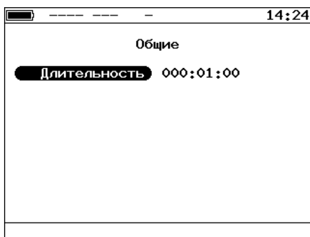
Рисунок 9.50. Меню «Общие»
