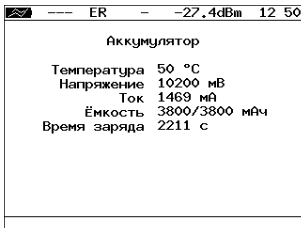
Рисунок 6.15. Экран «Аккумулятор»
