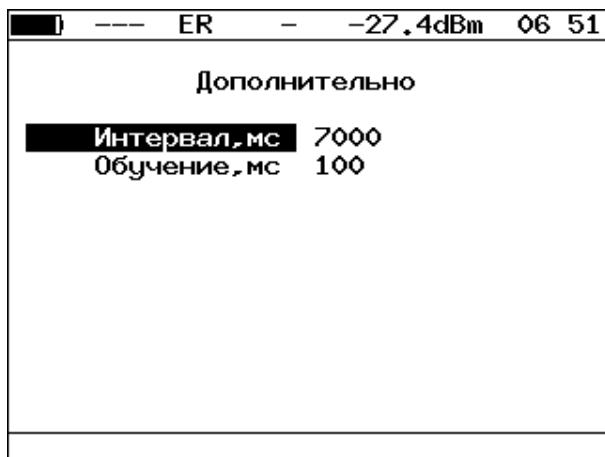
Рисунок 9.29. Меню «Дополнительно»
