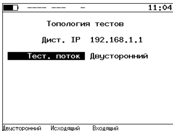
Рисунок 9.5. Меню «Топология»
