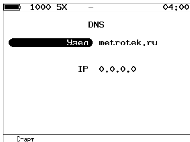
Рисунок 8.9. Меню «DNS»
