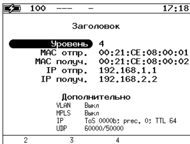
Рисунок 9.16. Меню «Заголовок»
