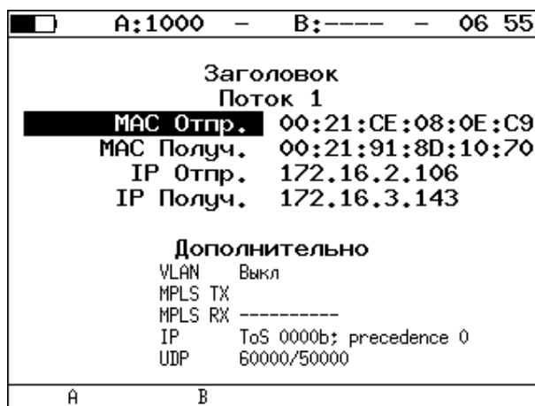
Рисунок 9.8. Экран «Заголовок»
