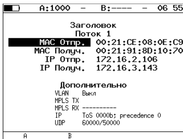
Рисунок 9.11. Экран «Заголовок»
