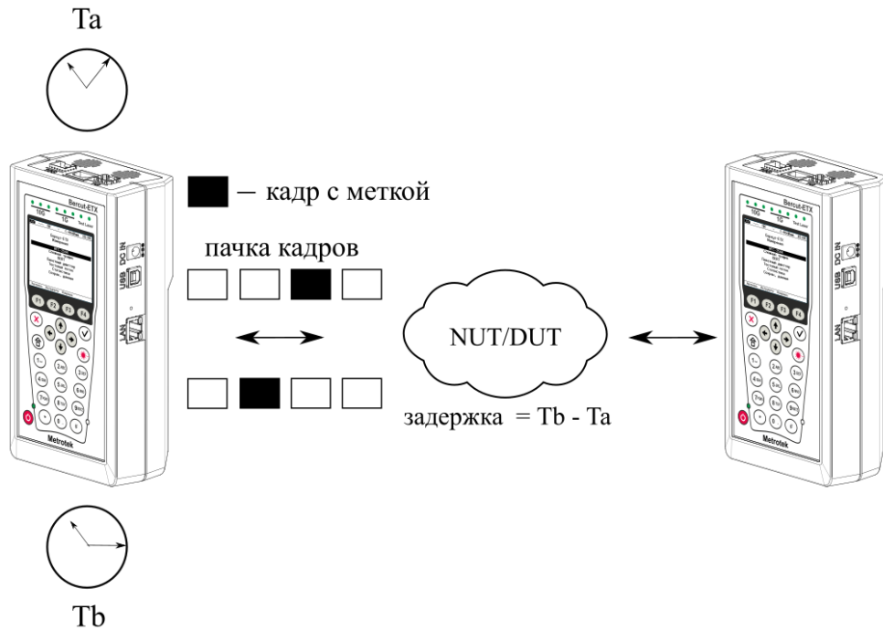
Рисунок 9.13. Анализ задержки
