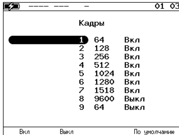
Рисунок 9.23. Меню «Кадры»
