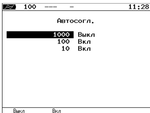
Рисунок 6.3. Меню «Автосогласование»
