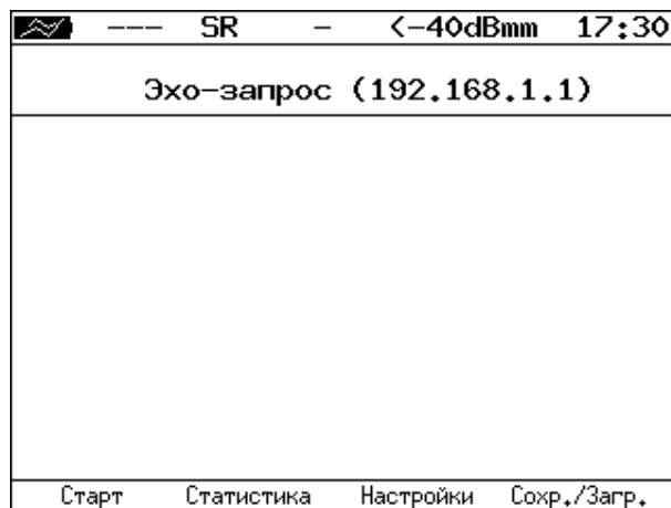
Рисунок 8.2. Меню «Эхо-запрос»
