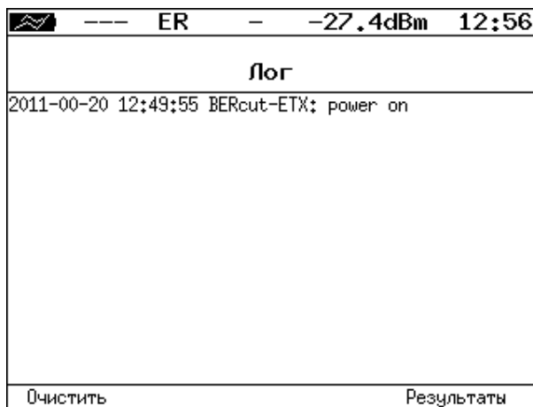
Рисунок 6.18. Меню «Лог»
