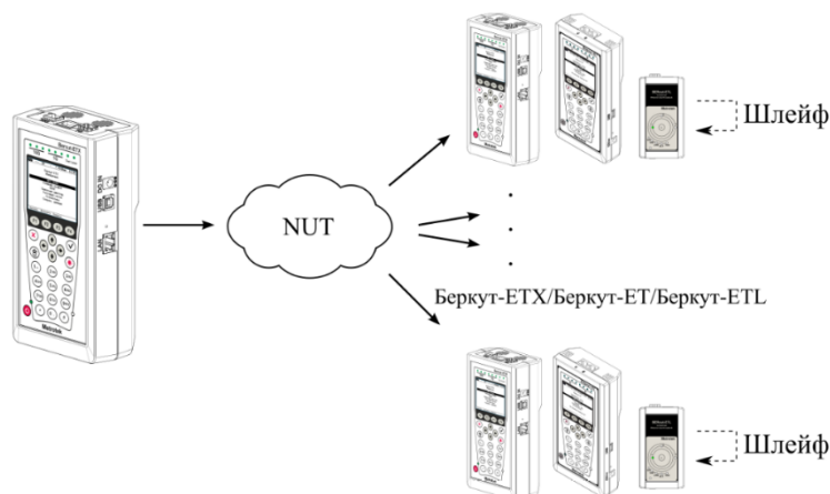
Рисунок 8.17. Схема тестирования
