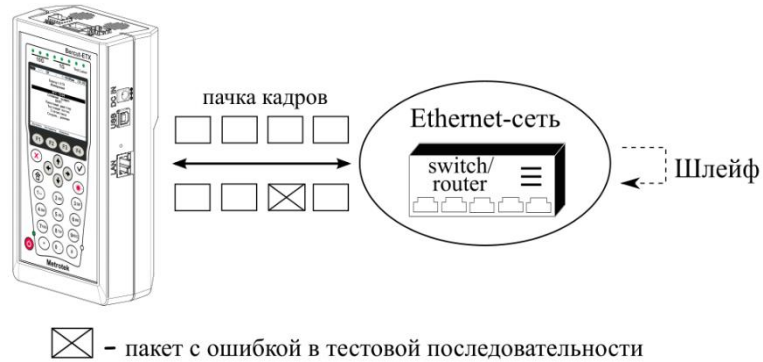
Рисунок 20.11. Тестирование на канальном/сетевом уровне (вариант 2)
