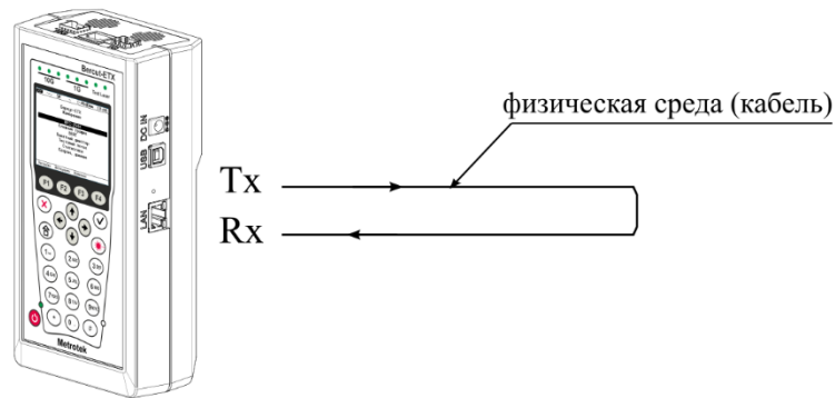
Рисунок 20.8. Тестирование на физическом уровне (вариант 1)
