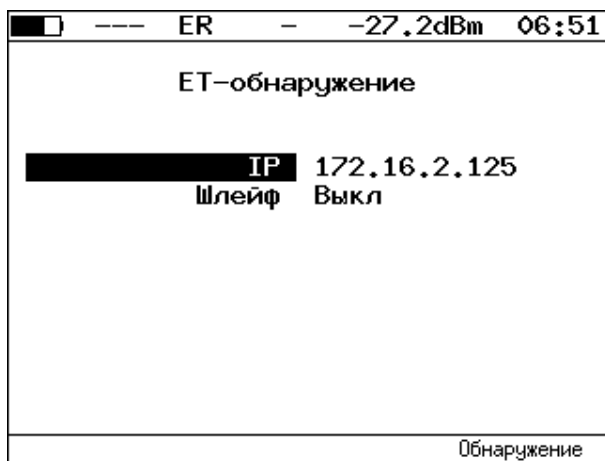
Рисунок 17.2. Меню «ET-обнаружение»
