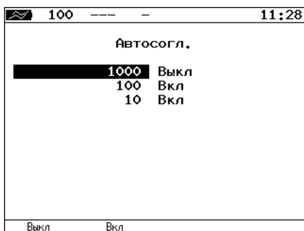
Рисунок 27.2. Меню «Автосогласование»
