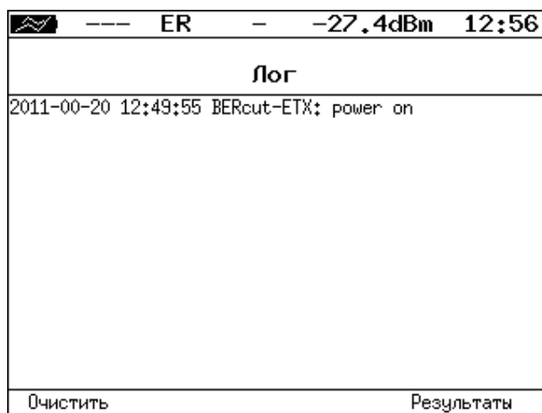
Рисунок 30.2. Меню «Лог»
