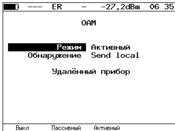
Рисунок 16.2. Меню «OAM»
