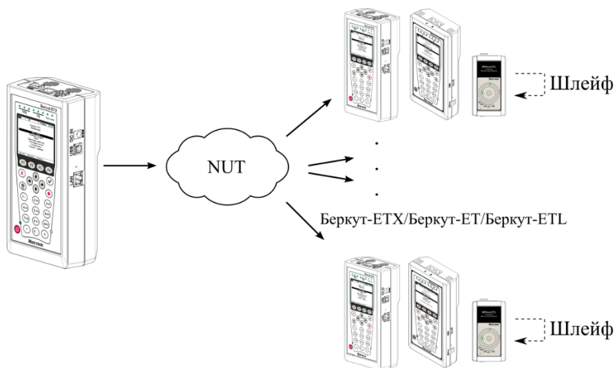
Рисунок 17.1. Схема тестирования
