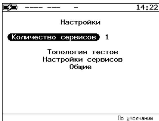
Рисунок 13.2. Меню «Настройки»
