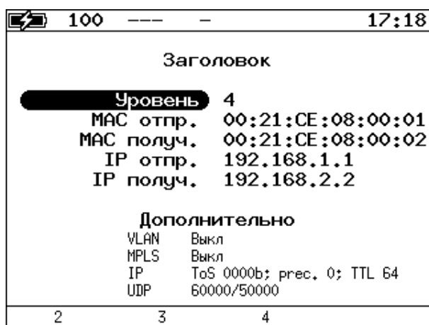
Рисунок 10.1. Меню «Заголовок»
