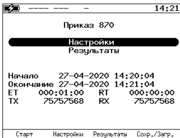
Рисунок 13.1. Меню «Приказ 870»
