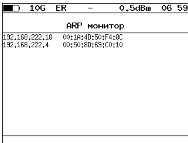
Рисунок 18.11. Результаты тестирования
