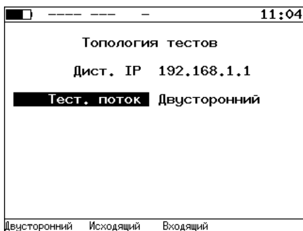
Рисунок 7.5. Меню «Топология»
