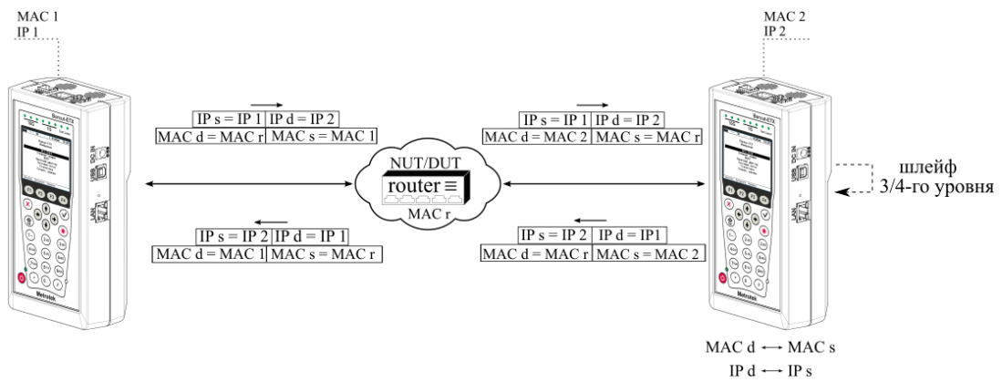
Рисунок 7.2. Типовая схема подключения 2
