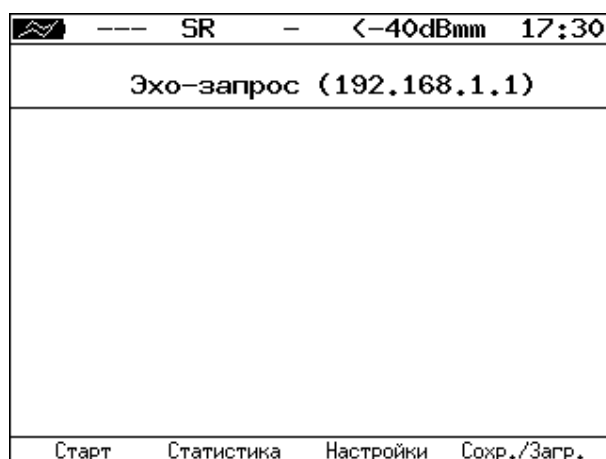
Рисунок 18.2. Меню «Эхо-запрос»
