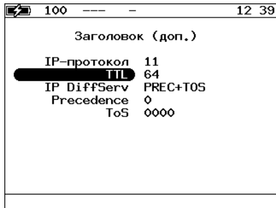
Рисунок 10.3. Настройка IP
