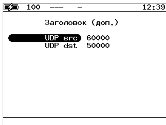
Рисунок 10.4. Настройка UDP
