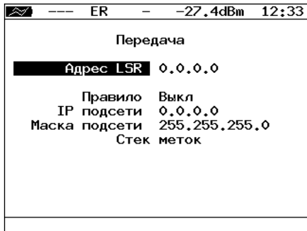
Рисунок 27.4. Меню «Передача»
