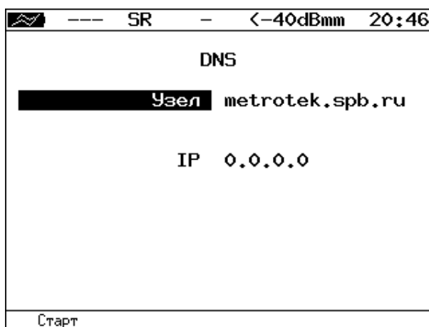
Рисунок 18.9. Меню «DNS»
