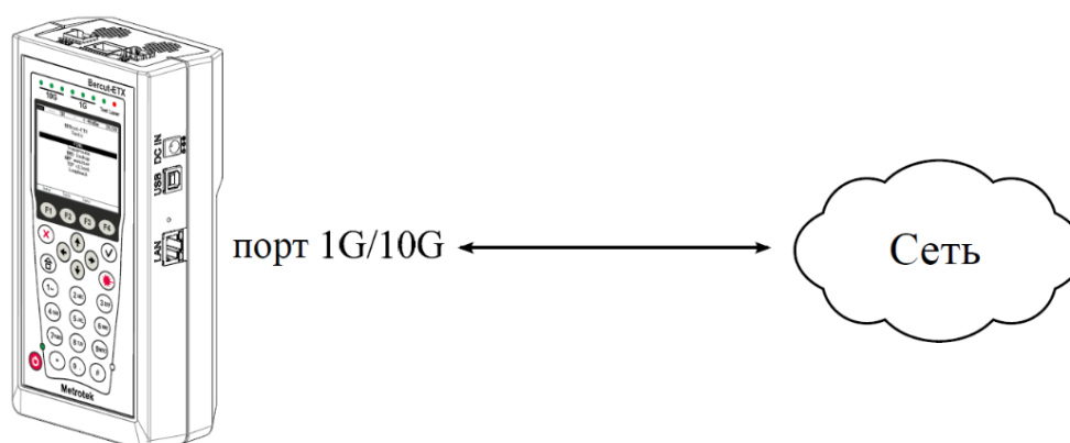
Рисунок 18.1. Схема подключения
