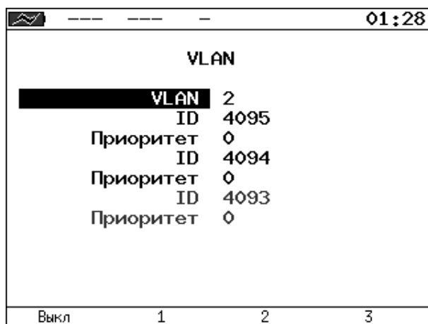
Рисунок 10.5. Меню «VLAN»
