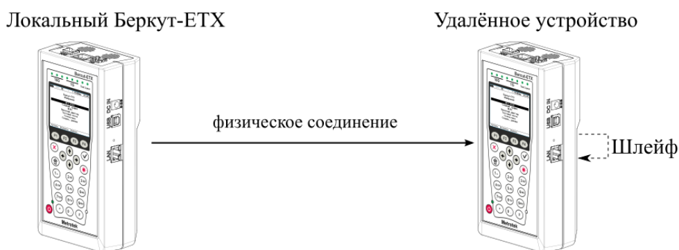
Рисунок 16.1. Схема тестирования
