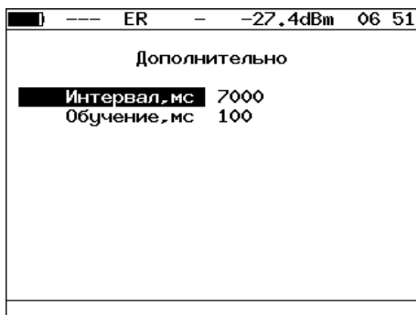
Рисунок 10.13. Меню «Дополнительно»
