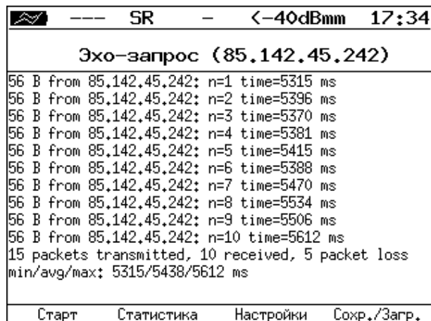
Рисунок 18.4. Результаты теста «Эхо-запрос»
