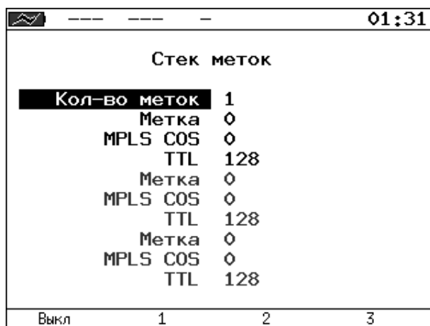
Рисунок 10.6. Меню «Стек меток»
