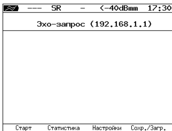
Рисунок 18.2. Меню «Эхо-запрос»
