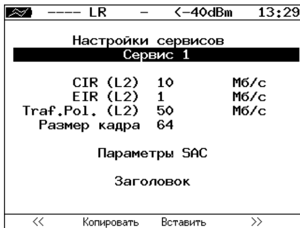
Рисунок 12.3. Меню «Y.1564. Настройки сервисов»
