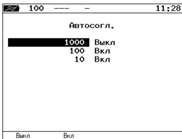
Рисунок 27.2. Меню «Автосогласование»
