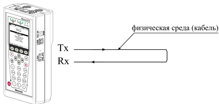
Рисунок 20.8. Тестирование на физическом уровне (вариант 1)
