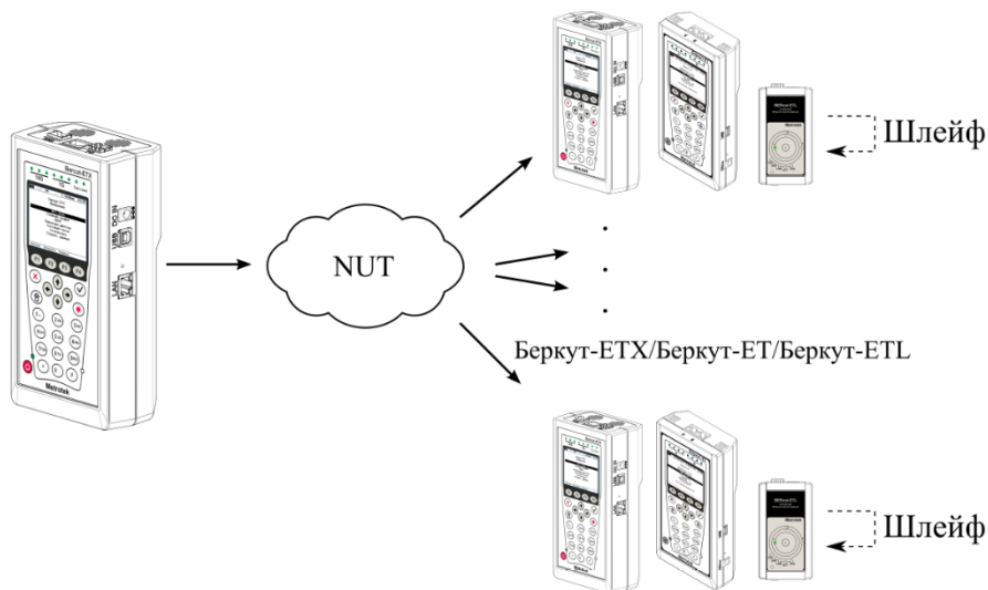
Рисунок 17.1. Схема тестирования
