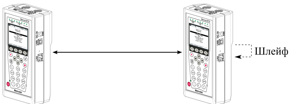
Рисунок 20.9. Тестирование на физическом уровне (вариант 2)
