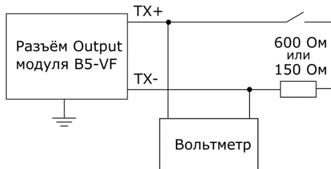
Рисунок 10.3. Схема подключения
