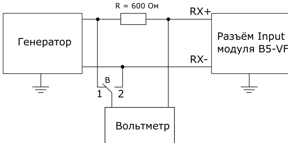
Рисунок 10.6. Схема подключения
