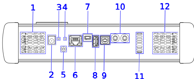
Рис. 5.2. Нижняя панель
