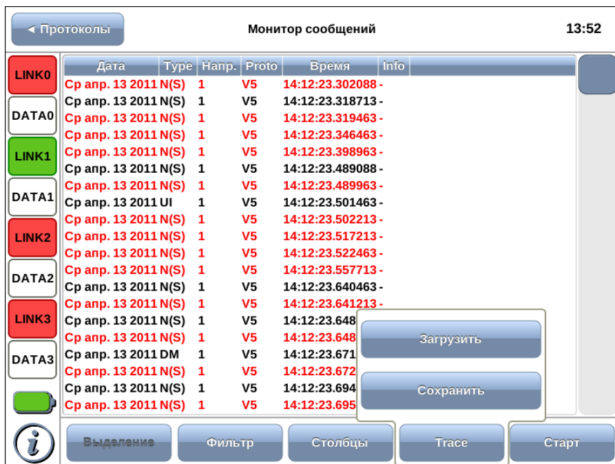
Рис. 9.1. Сохранение/загрузка трейс-файлов
