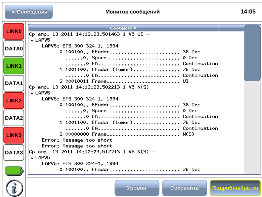
Рис. 9.4. Окно просмотра
