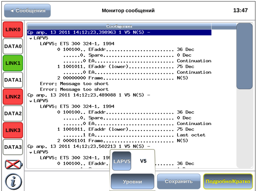
Рис. 7.7. Настройка уровней
