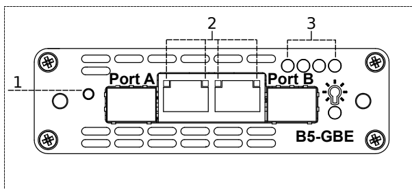
Рис. 5.1. Передняя панель модуля B5-GBE
