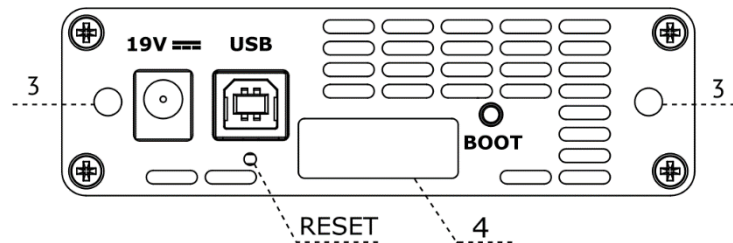
Рисунок 5.2. Задняя панель модуля B5-GBE
