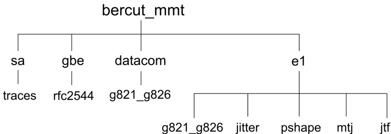
Рисунок 26.1. Структура каталогов
