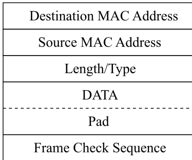
Рисунок 23.1. Структура Ethernet-кадра
