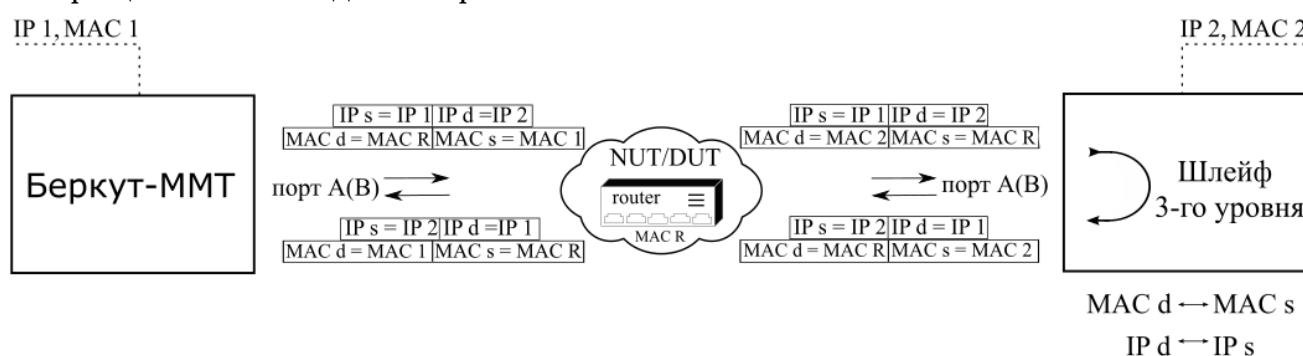
Рисунок 9.2. Вариант подключения 2
