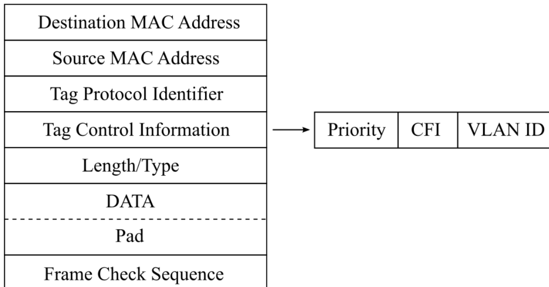
Рисунок 23.2. Структура Ethernet-кадра, содержащего VLAN-метку
