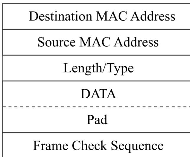
Рисунок 23.1. Структура Ethernet-кадра
