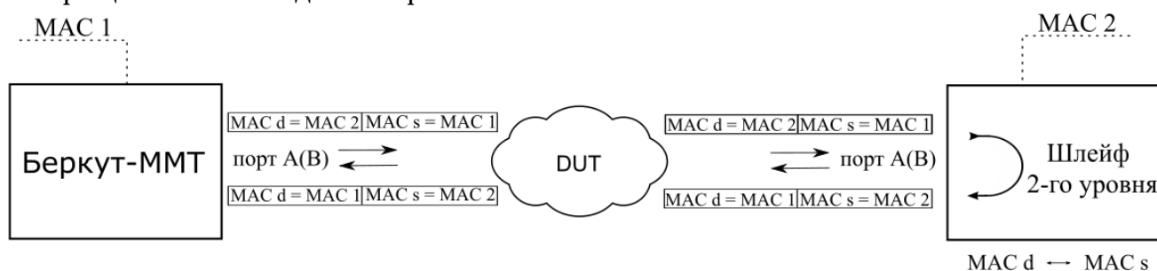
Рисунок 9.1. Вариант подключения 1
