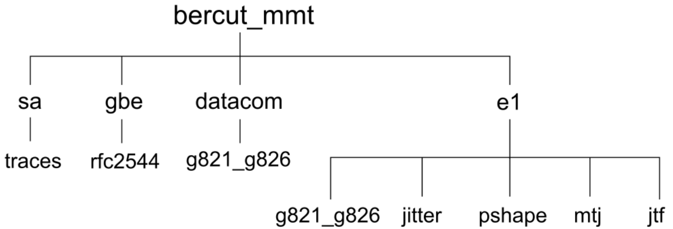
Рисунок 26.1. Структура каталогов
