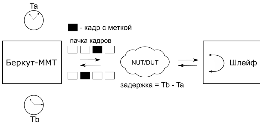
Рисунок 22.2. Анализ задержки
