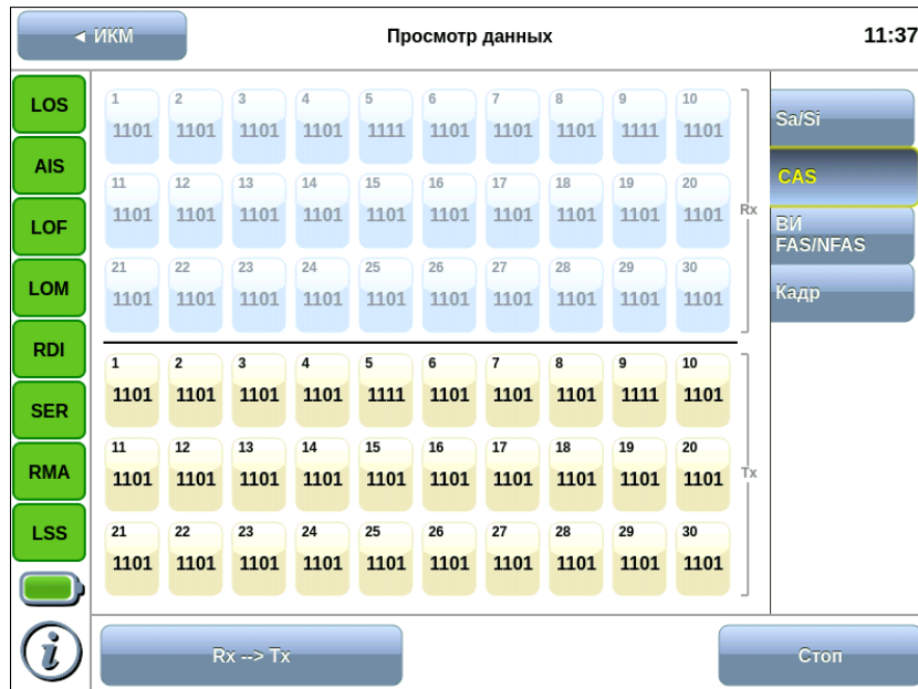
Рисунок 12.2. Вкладка «Сигнальные биты CAS», поток ИКМ30
