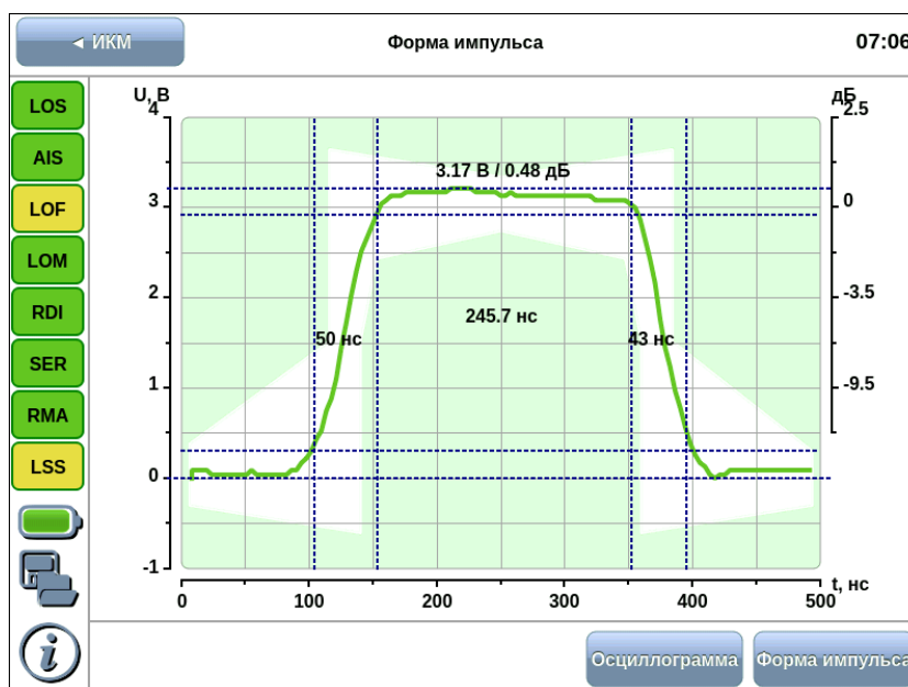
Рисунок 11.1. Приложение «E1 – Форма импульса»
