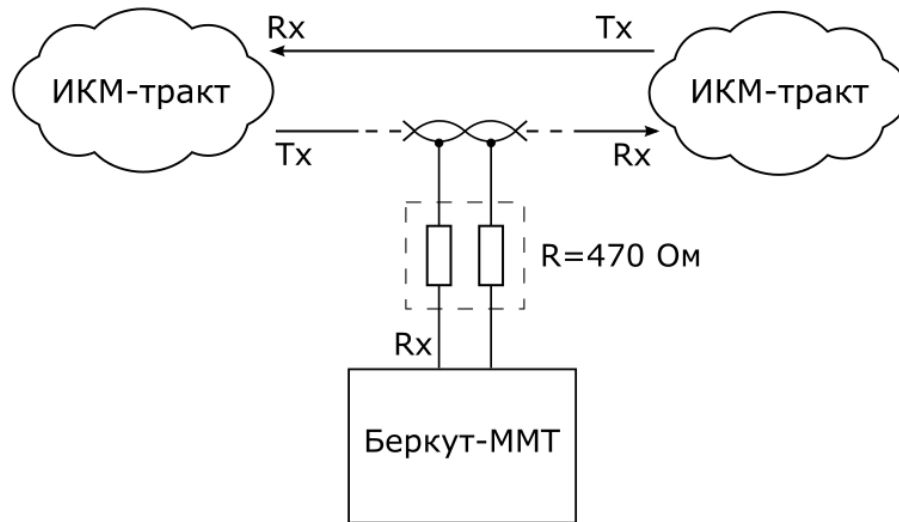
Рисунок 6.6. Использование защитных резисторов
