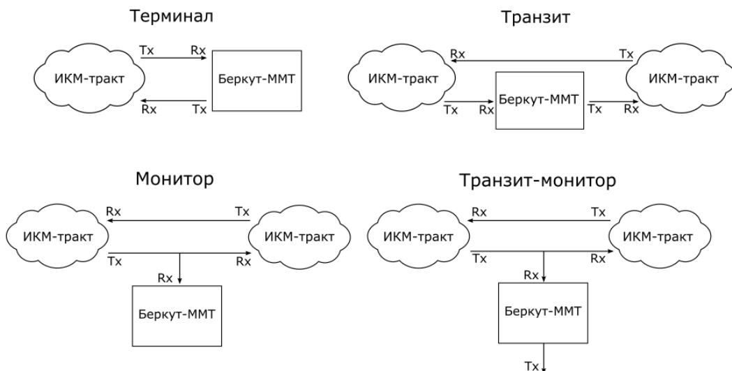
Рисунок 6.2. Режимы работы прибора
