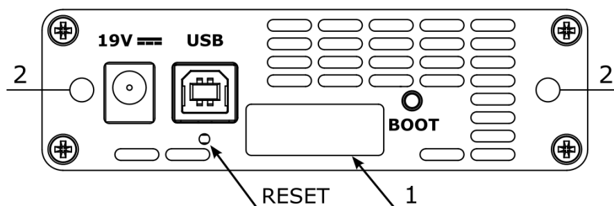
Рисунок 4.2. Задняя панель модуля E1
