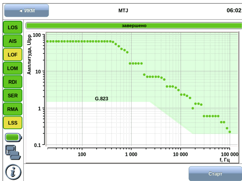
Рисунок 10.7. Результаты измерения МТJ
