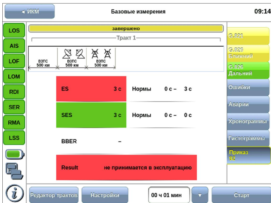
Рисунок 8.21. Результаты анализа в случае, когда тракт не прошел испытания
