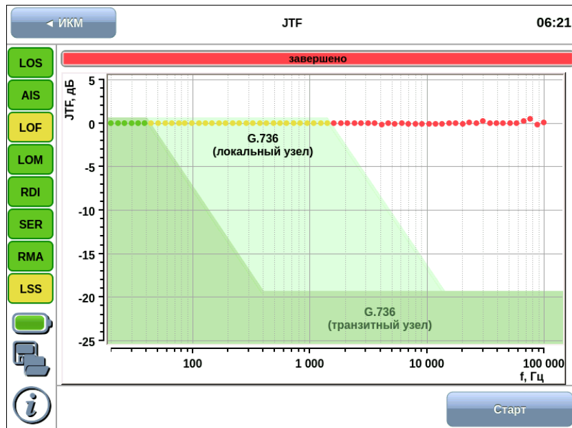
Рисунок 10.6. Результаты измерения JTF
