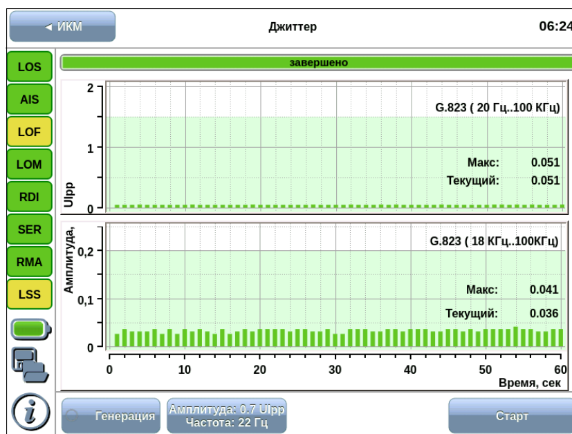
Рисунок 10.5. Результаты измерения джиттера
