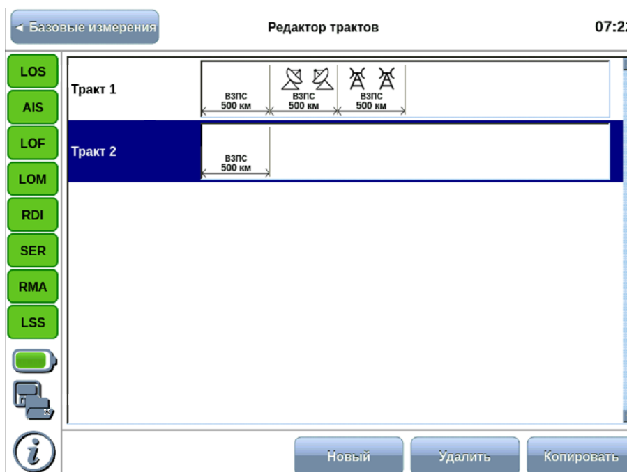
Рисунок 8.19. Приложение «Е1 – Редактор трактов»
