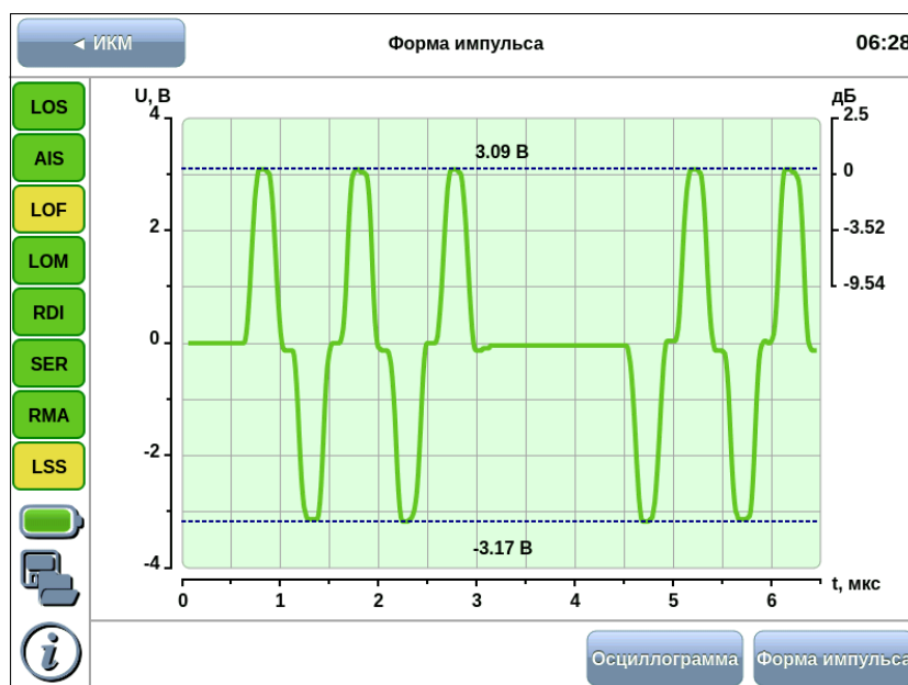
Рисунок 11.2. Отображение осциллограммы
