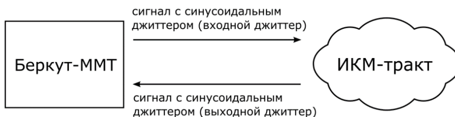
Рисунок 10.2. Измерение передаточной характеристики джиттера
