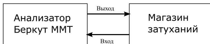
Рисунок 14.2. Определение чувствительности входа приёмника
