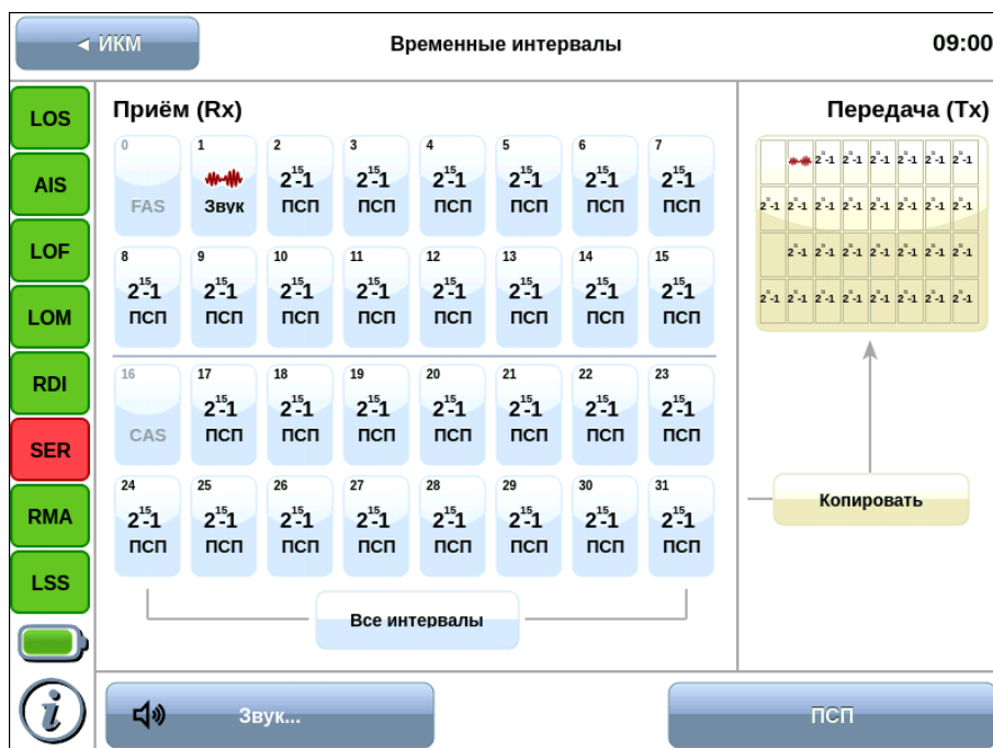
Рисунок 7.1. Приложение «Анализ E1 — Временные интервалы»
