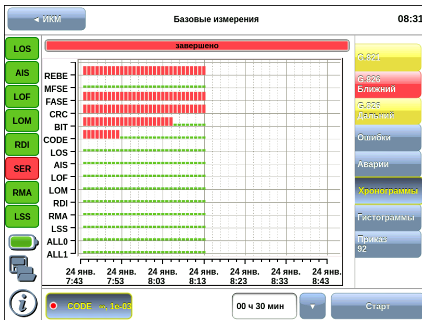
Рисунок 8.12. Вкладка «Хронограммы»
