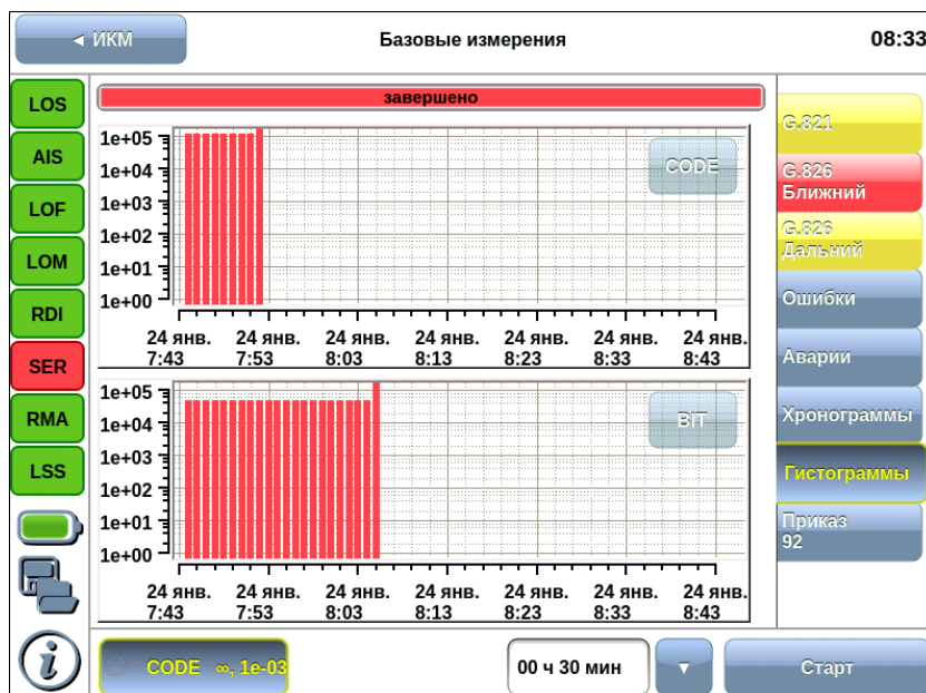
Рисунок 8.13. Вкладка «Гистограммы»
