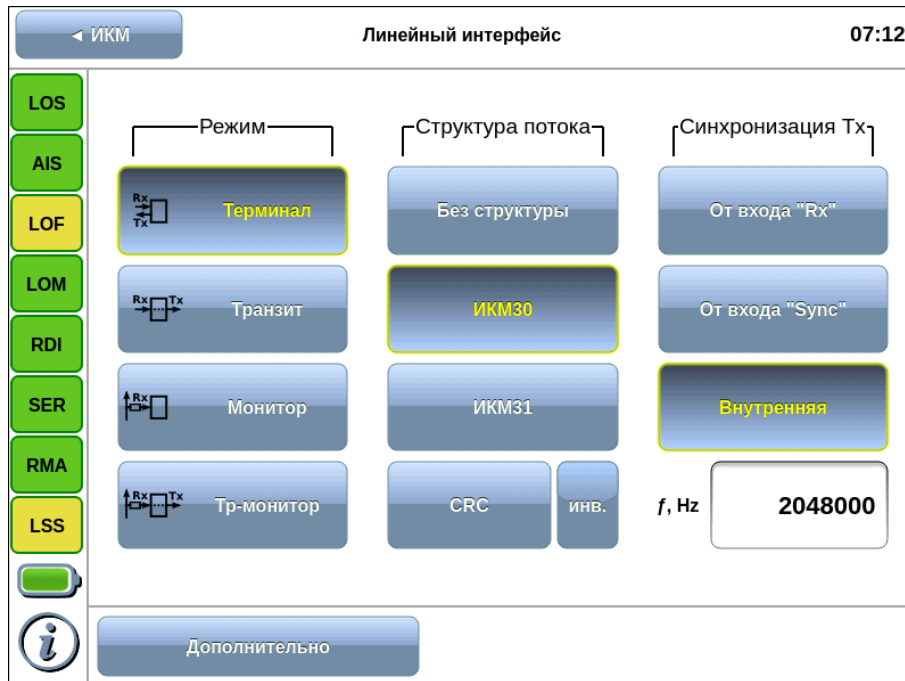
Рисунок 6.1. Приложение «E1 – Линейный интерфейс»
