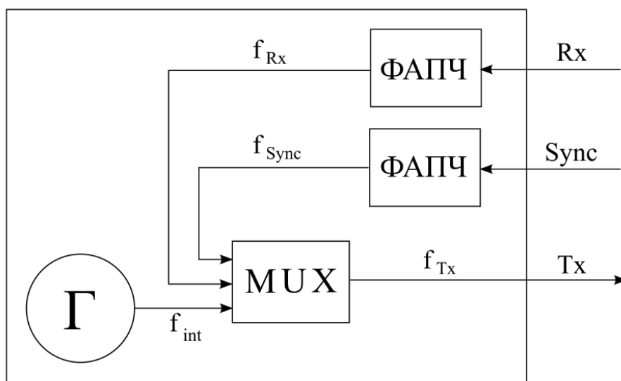
Рисунок 6.3. Схема мультиплексирования частоты передачи
