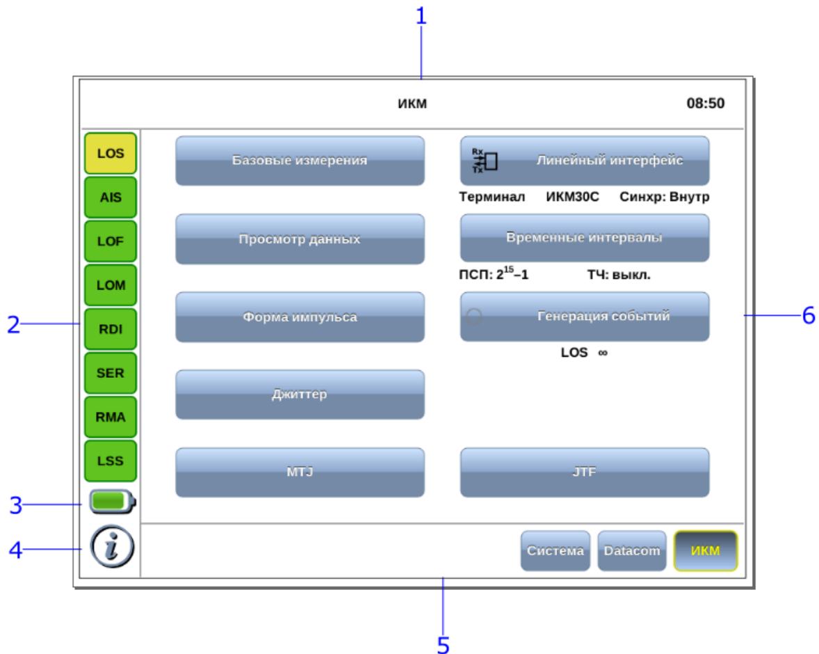
Рисунок 5.1. Главное меню
