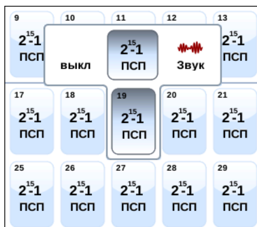
Рисунок 7.2. Диалоговое окно
