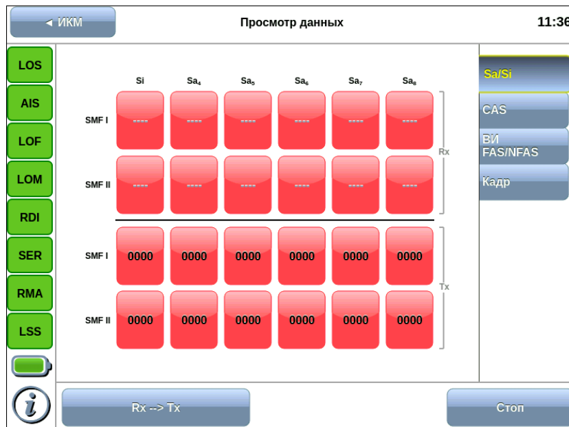
Рисунок 12.1. Вкладка Sa/Si
