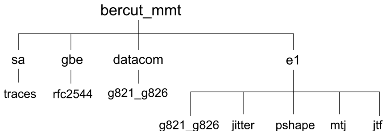
Рисунок 17.1. Структура каталогов
