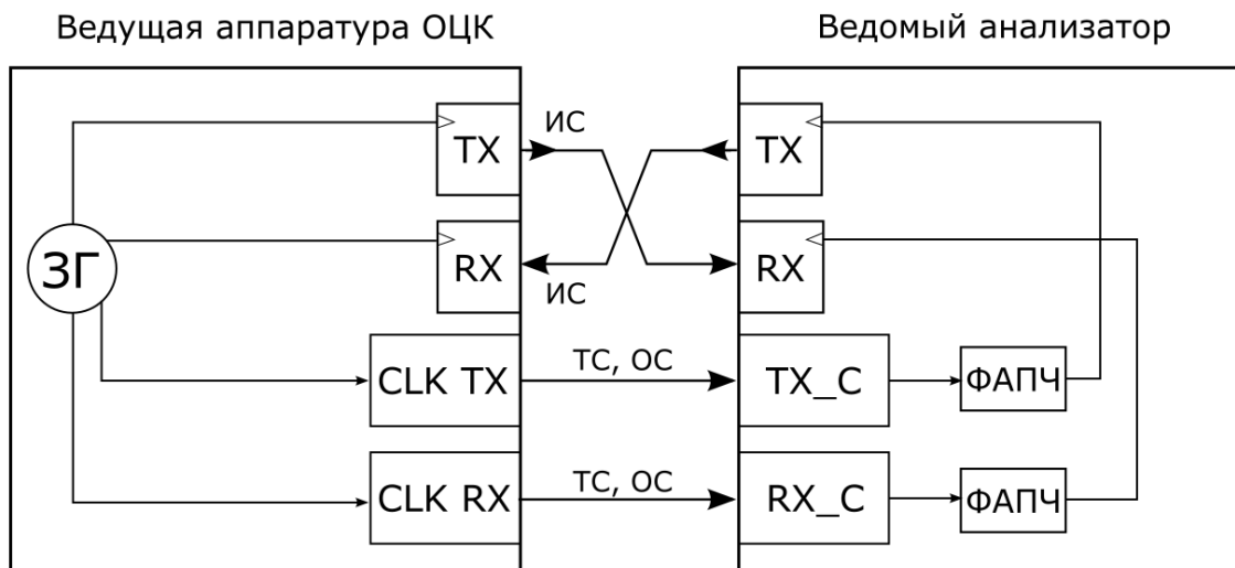
Рисунок 7.2. Сонаправленный стык: направление информационных (ИС), тактовых (ТС) и ответных сигналов (ОС)
