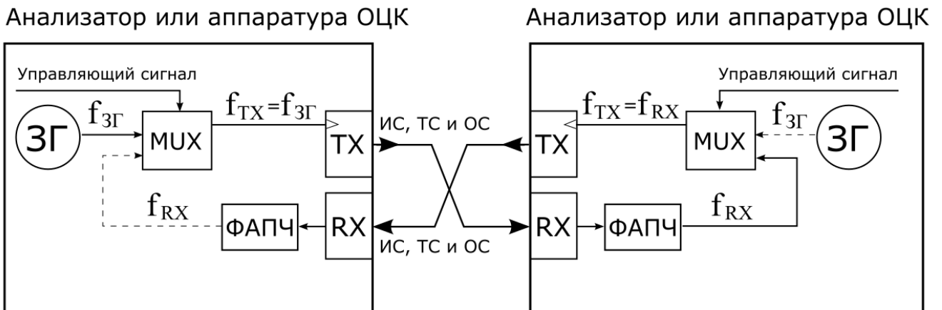
Рисунок 7.2. Сонаправленный стык: направление информационных (ИС), тактовых (ТС) и ответных сигналов (ОС)
