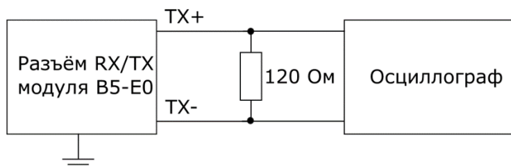
Рисунок 10.3. Схема подключения
