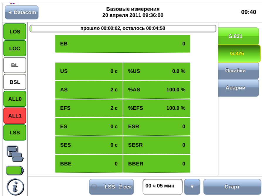
Рис. 8.3. Отчёт о проведённых измерениях
