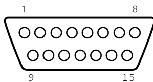
Рис. А.1. Интерфейс адаптера А1 (вилка)
