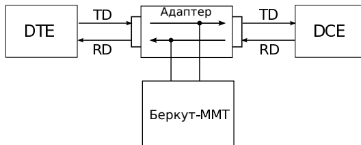
Рис. 7.4. Схема без вывода канала из обслуживания
