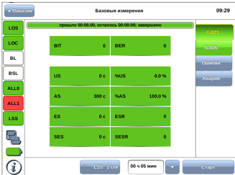
Рис. 7.6. Результаты измерений G.821
