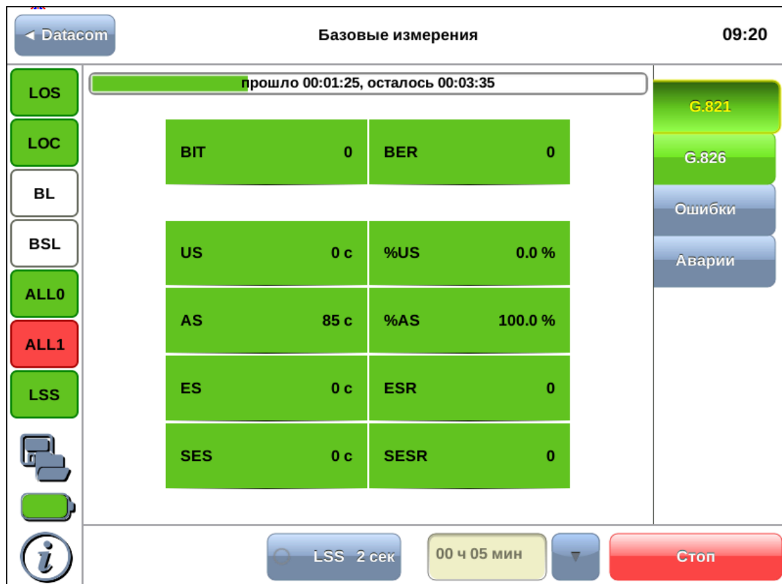
Рисунок 7.1. Приложение «DA – Базовые измерения»
