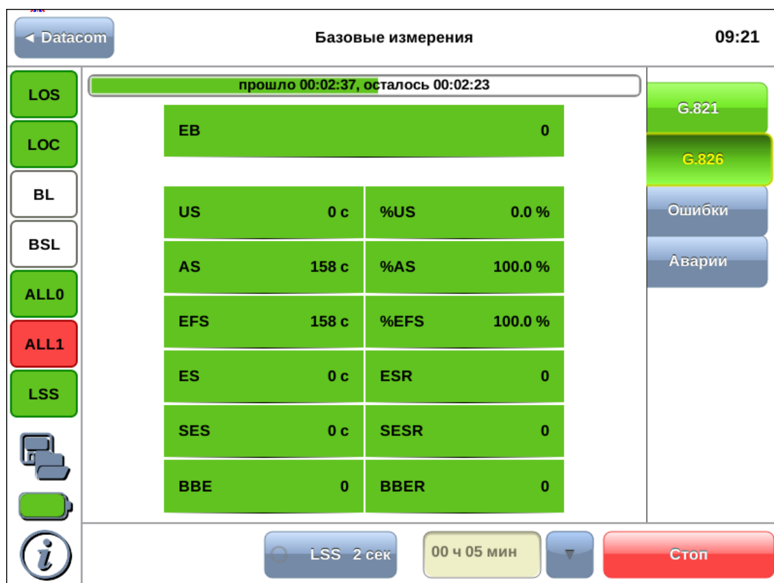
Рисунок 7.7. Результаты измерений G.826
