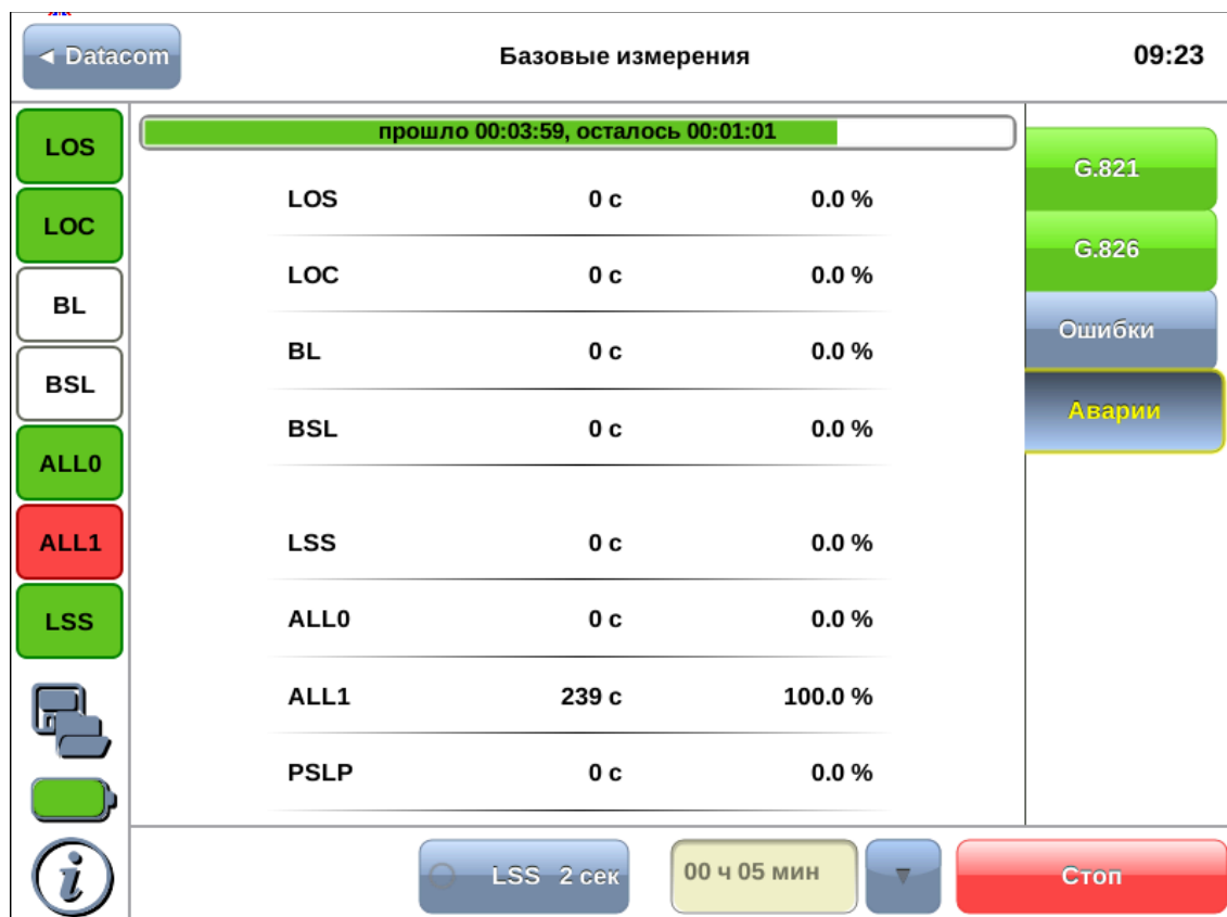
Рисунок 7.9. Вкладка «Аварии»
