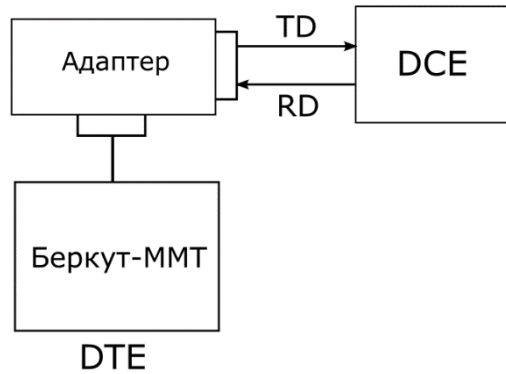
Рисунок 7.2. Схема с выводом канала из обслуживания. Вариант 1
