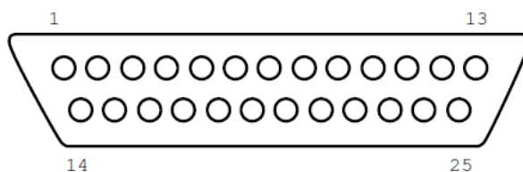
Рисунок 10.2. Интерфейс адаптера А2 (вилка)
