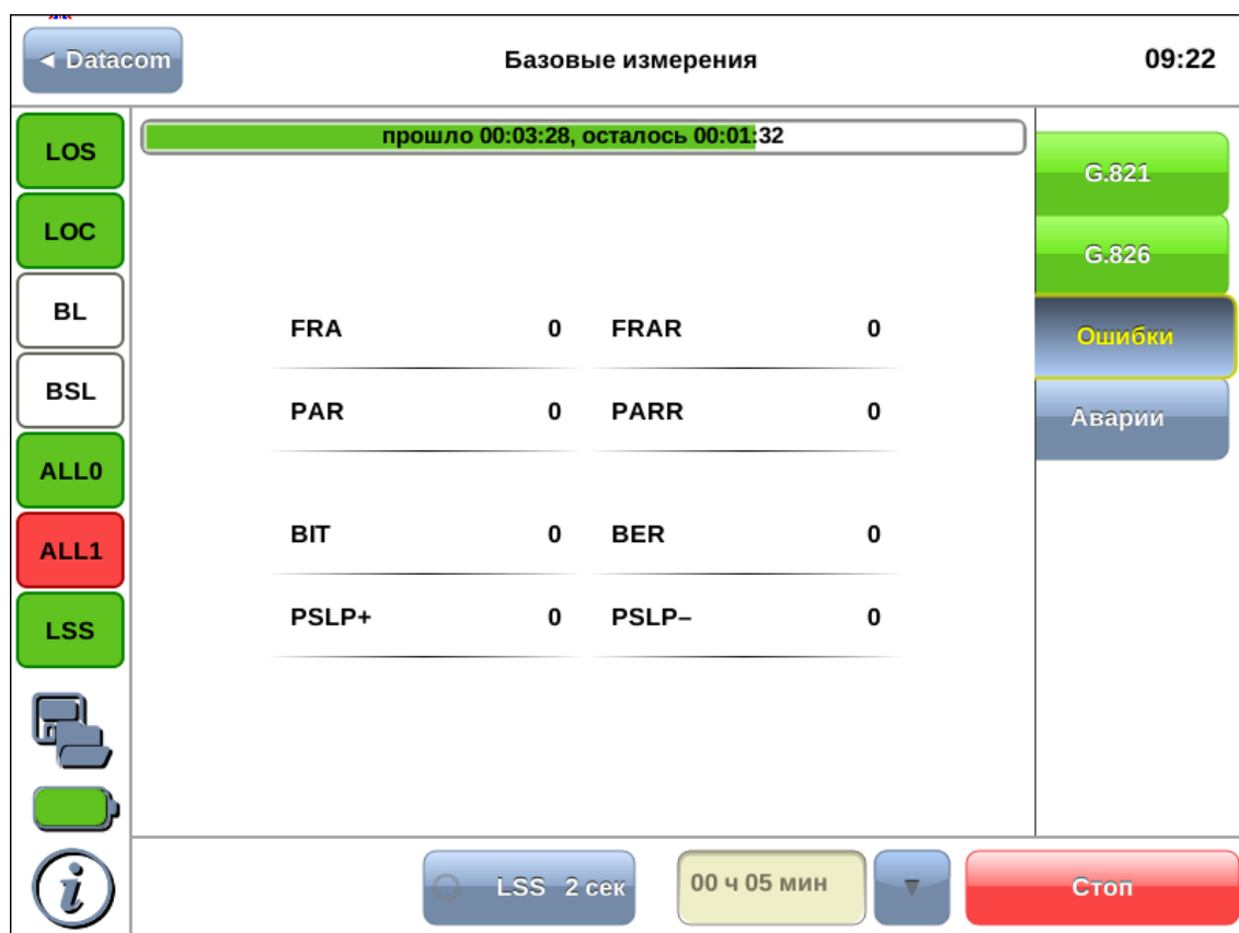
Рисунок 7.8. Вкладка «Ошибки»
