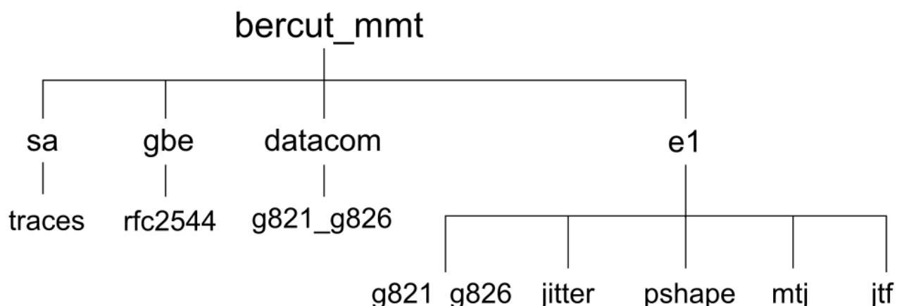
Рисунок 13.1. Структура каталогов
