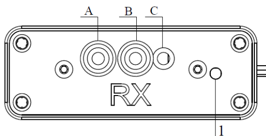
Рисунок 11.5. Интерфейс адаптера С1-И (приёмная часть)
