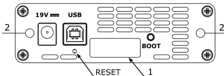
Рисунок 4.2. Задняя панель модуля B5-DA
