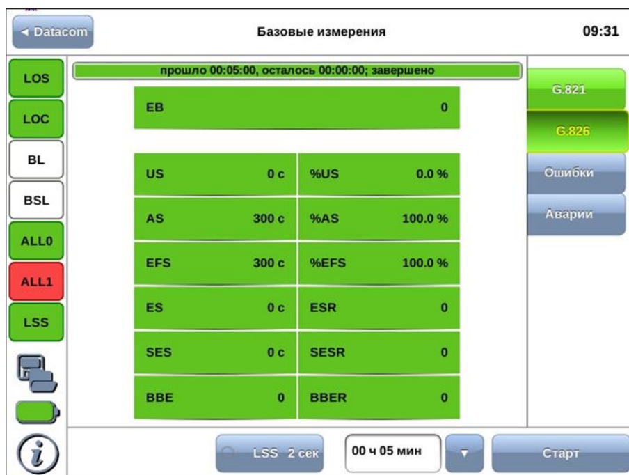
Рисунок 9.5. Результаты тестирования
