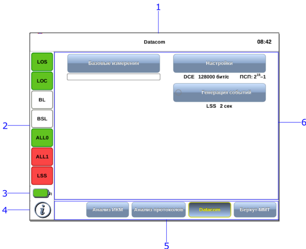
Рисунок 5.1. Главное меню
