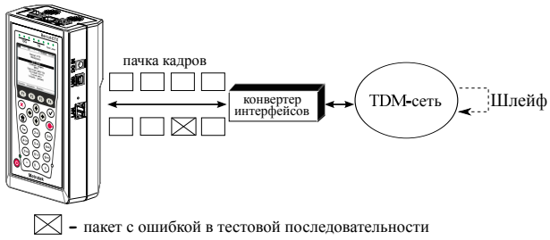
Рис. 17.12. Тестирование на канальном/сетевом уровне (вариант 3)
