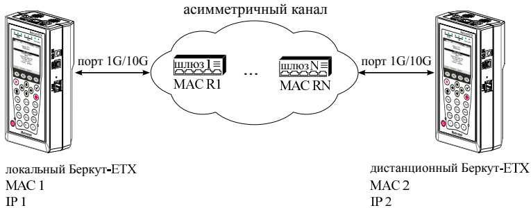
Рис. 10.2. Типовая схема подключения
