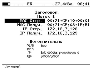
Рис. 11.7. Меню «Заголовок»
