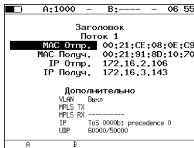
Рис. 10.3. Экран «Заголовок»
