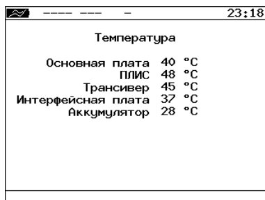
Рис. 24.5. Меню «Температура»
