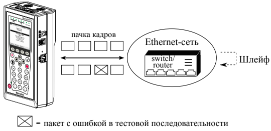
Рис. 17.11. Тестирование на канальном/сетевом уровне (вариант 2)
