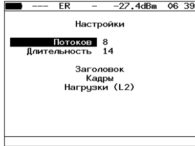
Рис. 11.6. Меню «Настройки»
