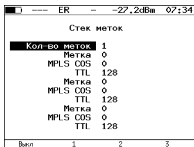
Рис. 17.7. Меню «MPLS»
