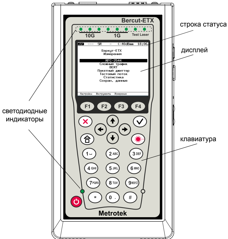
Рис. 5.1. Лицевая панель
