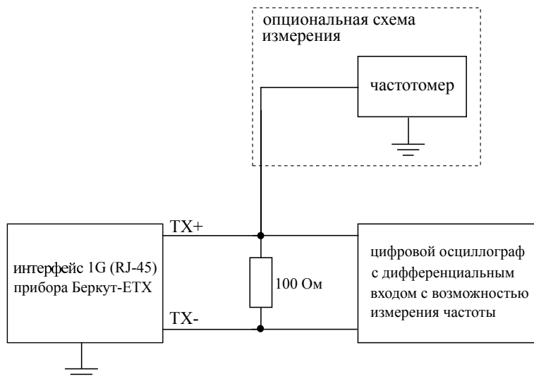
Рис. 29.1. Схема подключения
