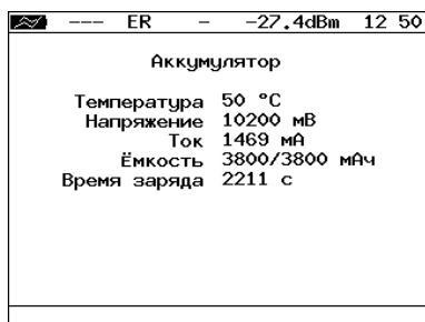
Рис. 24.4. Экран «Аккумулятор»
