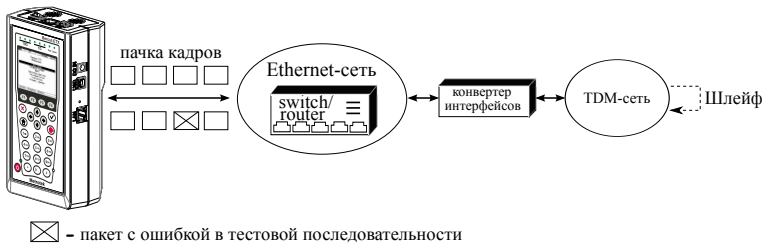
Рис. 17.10. Тестирование на канальном/сетевом уровне (вариант 1)
