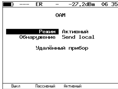
Рис. 13.2. Меню «OAM»
