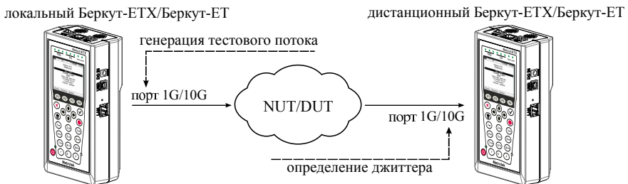
Рис. 19.3. Генерация постоянного трафика. Схема 2
