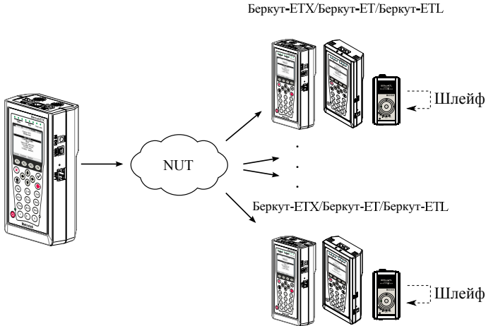
Рис. 14.1. Схема тестирования
