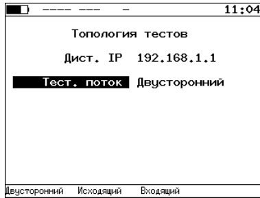
Рис. 7.3. Меню Топология
