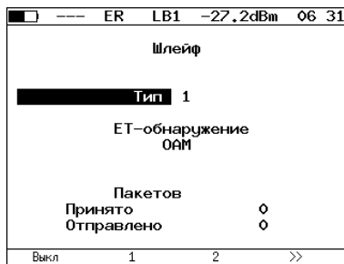
Рис. 12.1. Меню «Шлейф»
