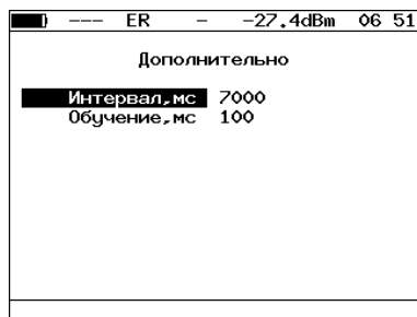
Рис. 7.14. Меню «Дополнительно»
