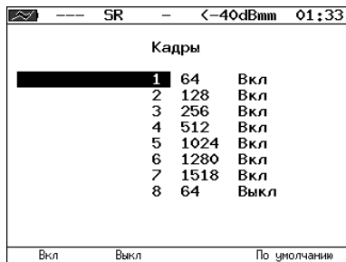
Рис. 7.8. Меню «Кадры»
