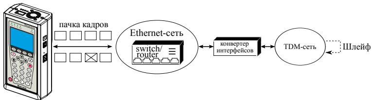
Рис. 14.10. Тестирование на канальном/сетевом уровне (вариант 1)
