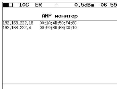
Рис. 13.11. Результаты тестирования
