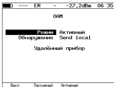
Рис. 11.2. Меню «ОАМ»
