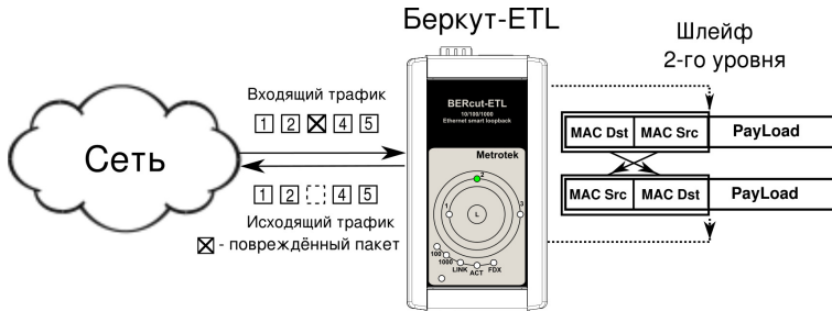
Рис. 4.2. Подключение шлейфа 2-го уровня
