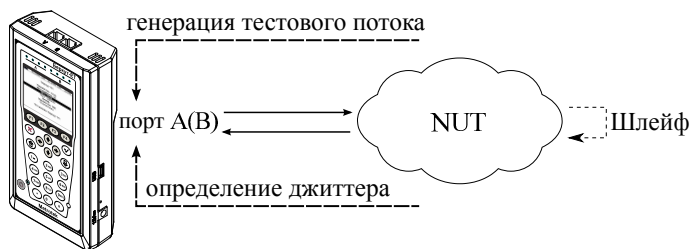
Рис. 7.109. Измерение джиттера. Схема 1
