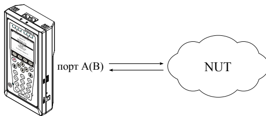
Рис. 7.72. Вариант подключения 1
