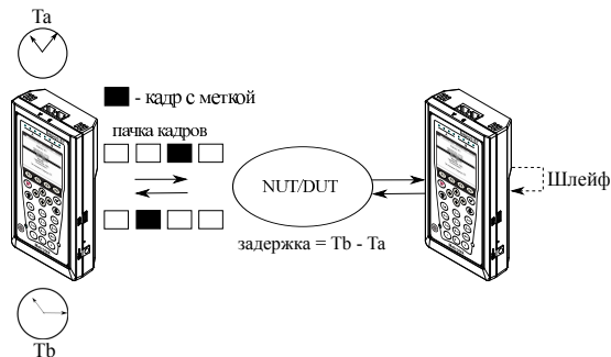
Рис. 7.2. Анализ задержки
