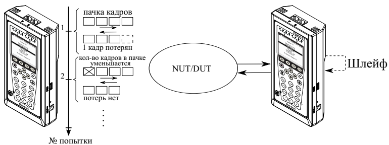
Рис. 7.4. Анализ предельной нагрузки
