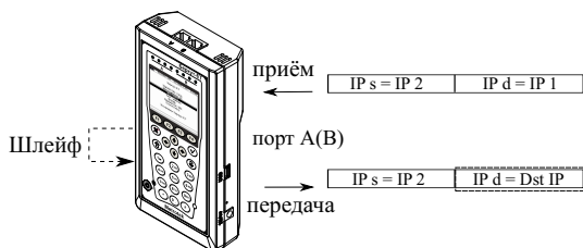
Рис. 7.52. Режим замены «Получ.»
