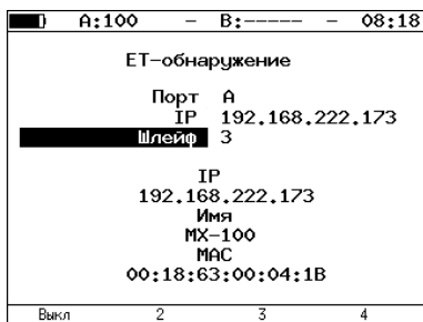
Рис. 7.59. Пример выполнения ЕТ-обнаружения
