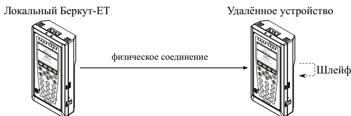
Рис. 7.54. Схема тестирования
