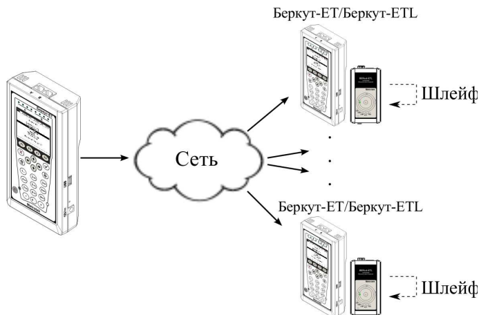
Рис. 7.57. Схема тестирования
