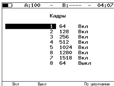
Рис. 7.18. Меню «Кадры»
