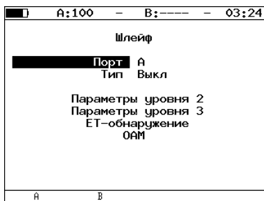
Рис. 7.45. Меню «Шлейф»
