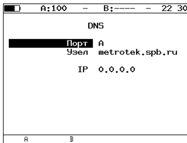
Рис. 7.69. Меню «DNS»
