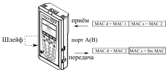
Рис. 7.48. Режим замены «Отпр.»
