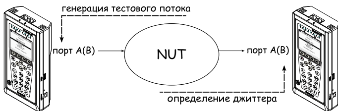
Рис. 7.89. Измерение джиттера. Схема 3
