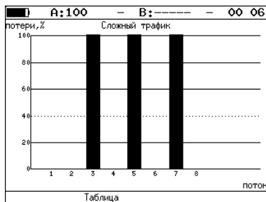
Рис. 7.32. Экран «Сложный трафик» (график)
