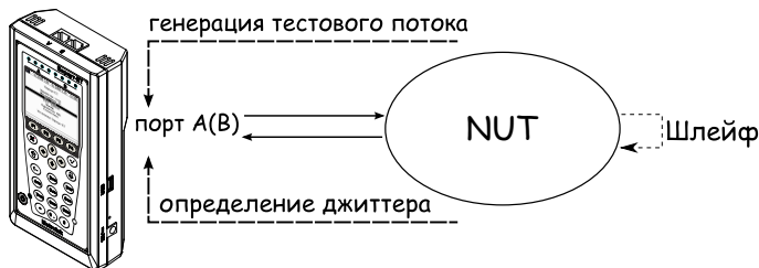
Рис. 7.87. Измерение джиттера. Схема 1
