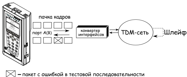
Рис. 7.82. Тестирование на канальном/сетевом уровне (вариант 3)
