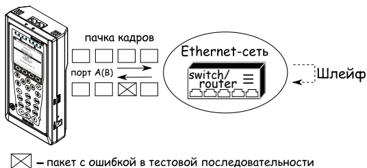
Рис. 7.81. Тестирование на канальном/сетевом уровне (вариант 2)
