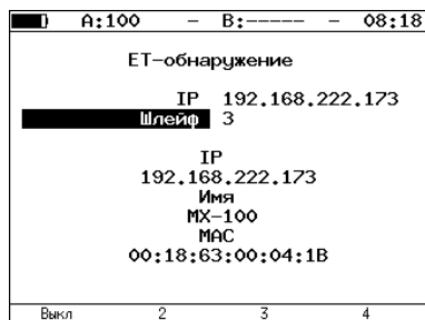
Рис. 7.55. Пример выполнения ЕТ-обнаружения
