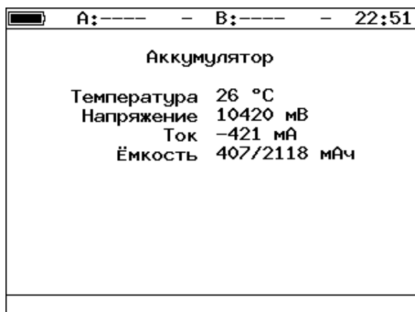
Рисунок 6.26. Экран «Аккумулятор»
