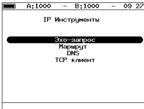
Рисунок 7.1. Меню «IP-инструменты»
