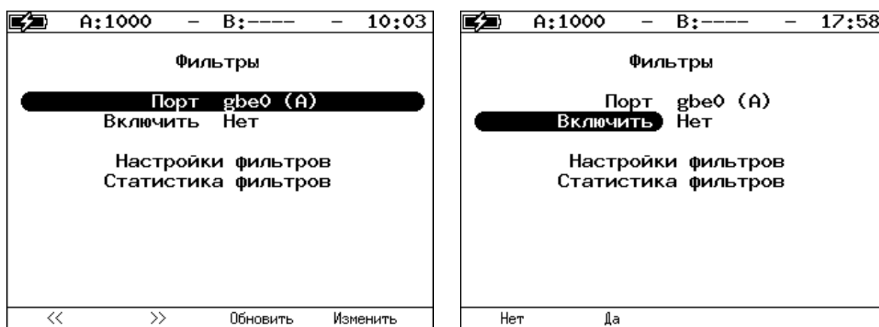
Рисунок 7.33. Меню «Фильтры»
