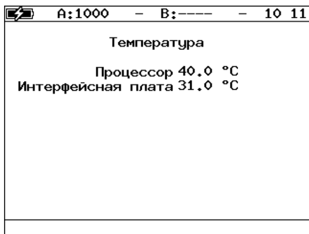
Рисунок 6.22. Экран «Температура»
