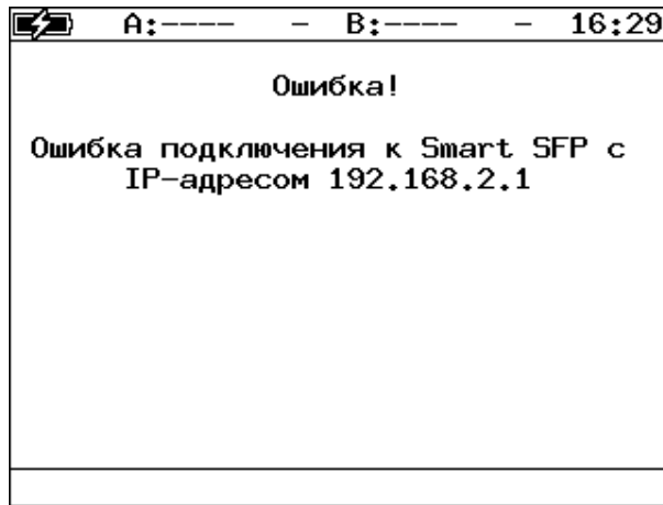
Рисунок 7.23. Ошибка подключения
