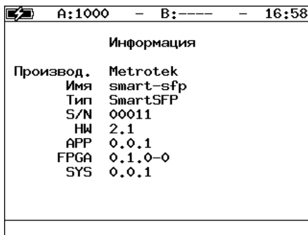
Рисунок 7.24. Меню «Информация»
